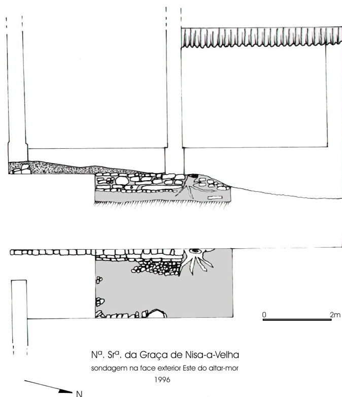
N. Sr.ª da Graça (14.14) - Imagem gentilmente cedida por Jorge de Oliveira: planta e alçado finais da sondagem arqueológica realizada em 1996 na face exterior Este do altar-mor da igreja, mostrando o aparelho construtivo (romano?) detectado sob a estrutura medieval.
