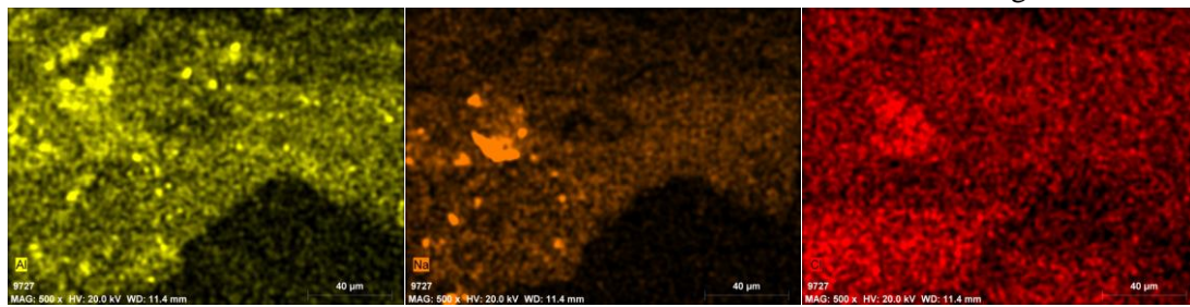
Al
