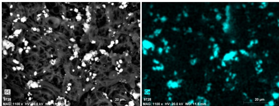
BSE
