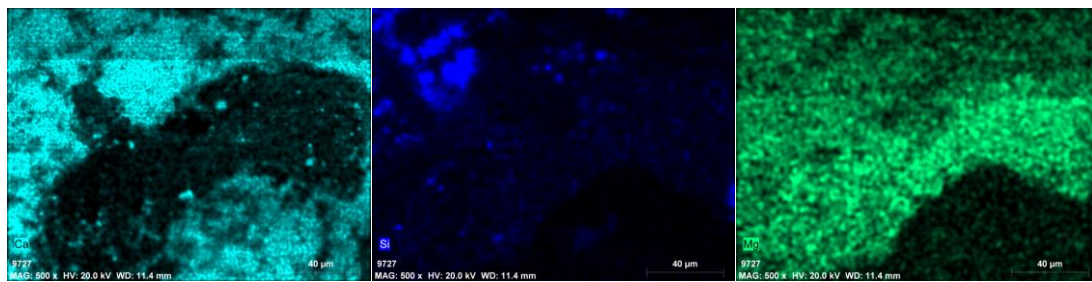
Ca
