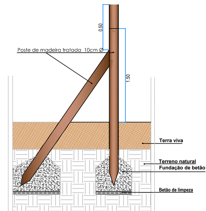
P - PORMENOR DO SISTEMA DE TRAVAMENTO DA VEDAÇÃO NOS CANTOS
