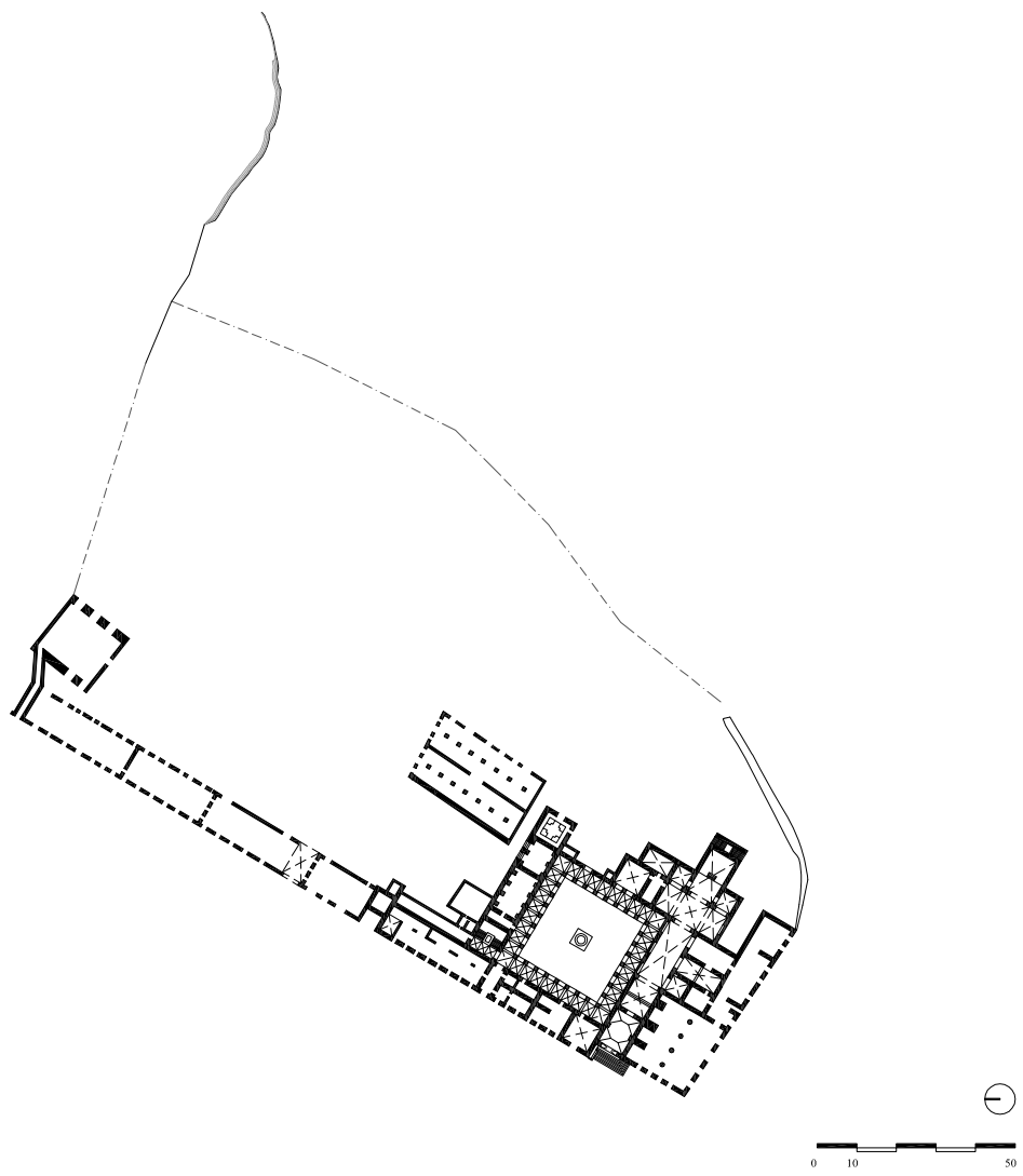
Fig. 1-c - Planta Convento de S. Francisco de Portalegre-séc. XIII, Portugal
