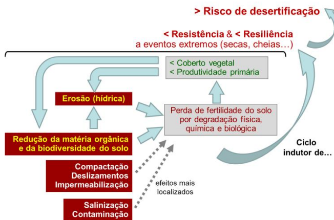
Figura 1: Os processos de degradação do solo diminuem a sua capacidade para sustentar a produção primária e, gradualmente, reduzem a resistência e a resiliência dos ecossistemas a eventos extremos.
