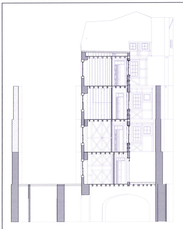
Corte A1, Escala 1:200
