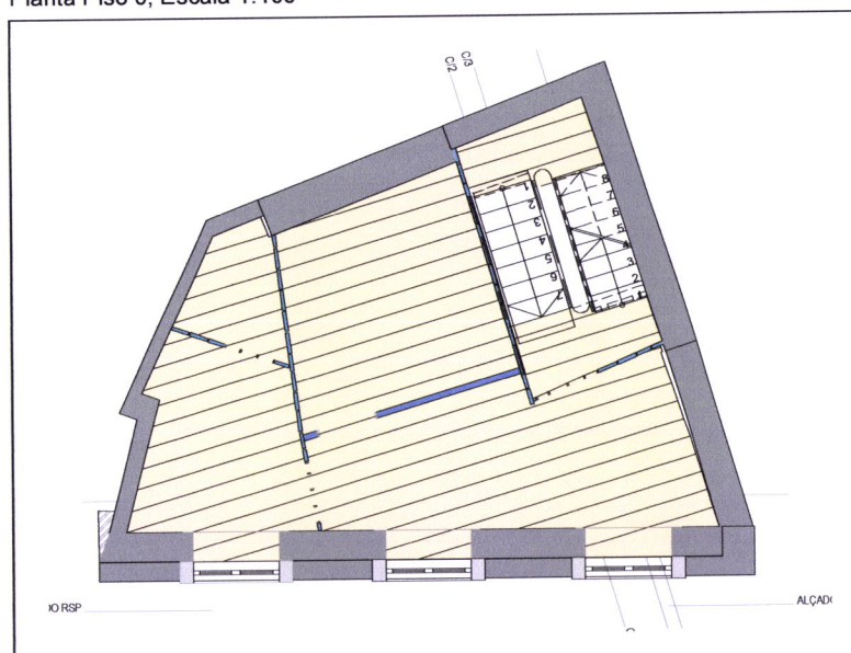
Planta Piso 1, Escala 1:100
