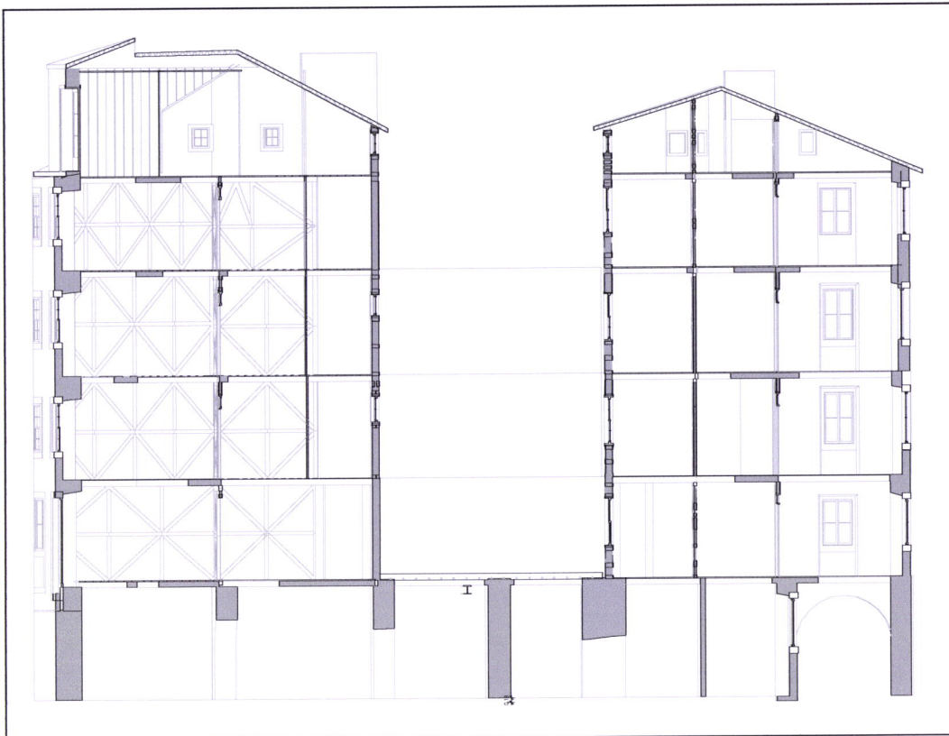
Corte B1, Escala 1:200
