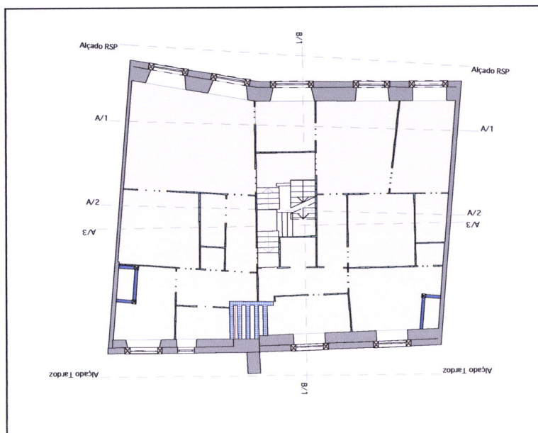
Planta Piso 2 , Escala 1:200
