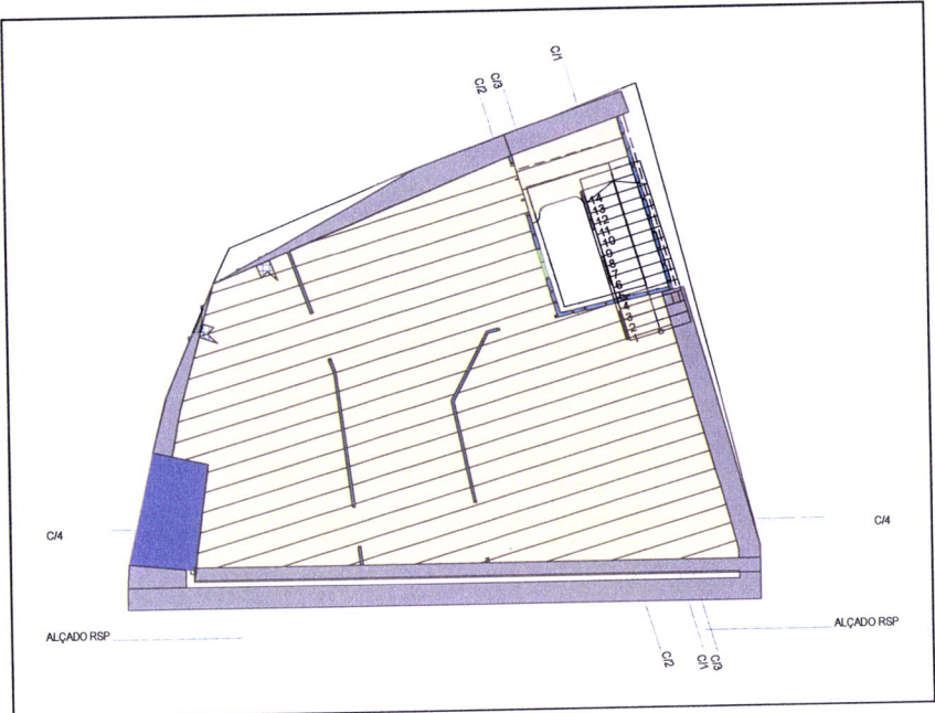
Planta Piso 3, Escala 1:100
