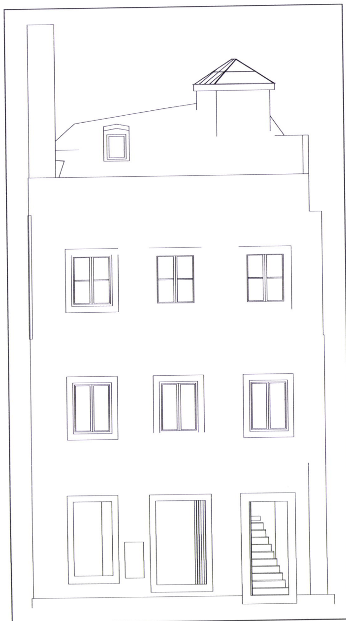
Alçado Rua de São Pedro, Escala 1:100
