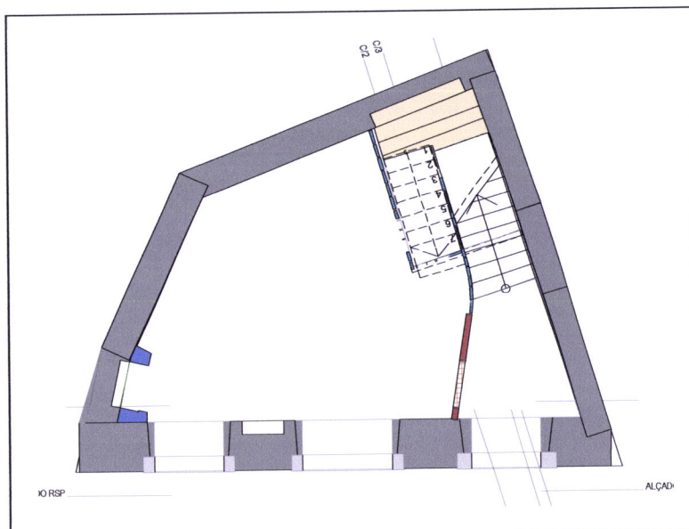
Planta Piso 0, Escala 1:100
