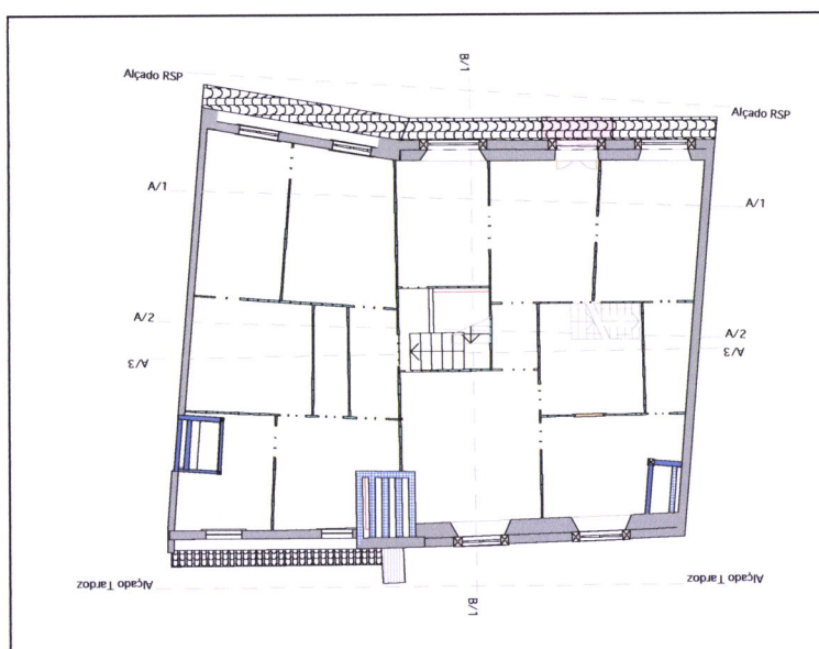
Planta Piso 3, Escala 1:200
