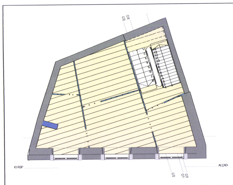
Planta Piso 2, Escala 1:100
