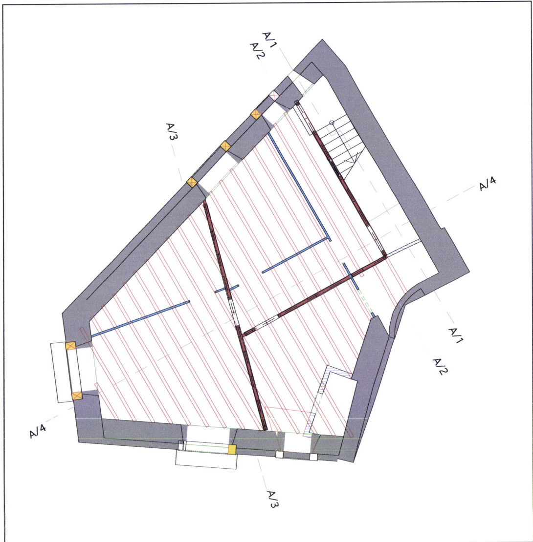
Planta Piso 2, Escala 1:100
