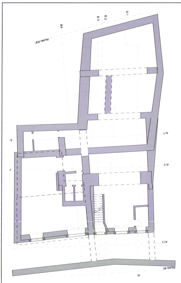
Planta Piso 0, Escala 1:200
