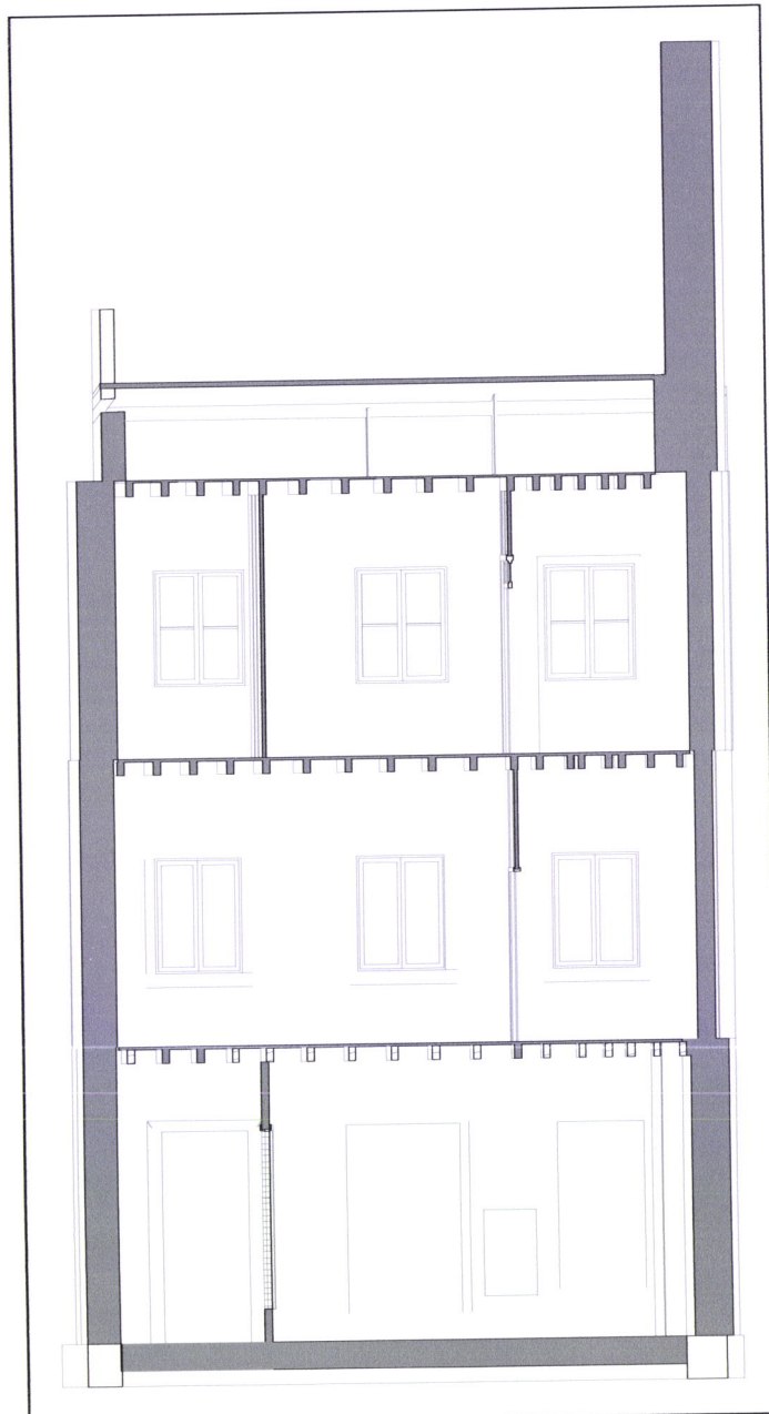
Corte 4, Escala 1:100
