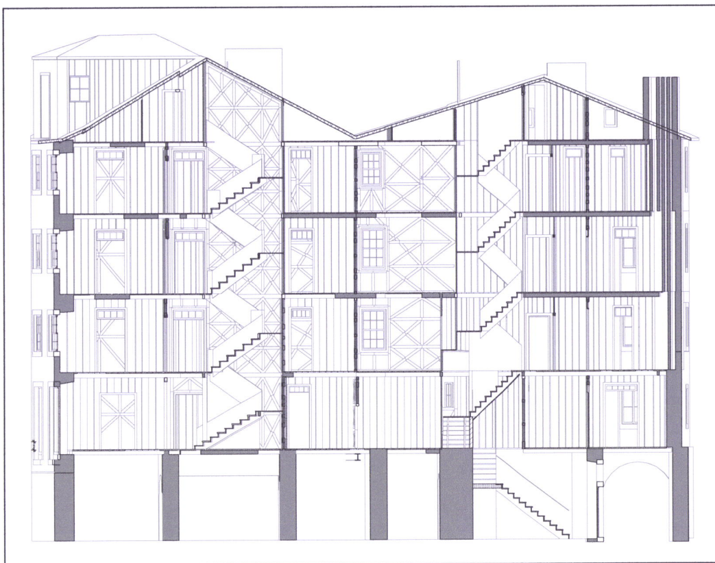
Corte B3, Escala 1:200
