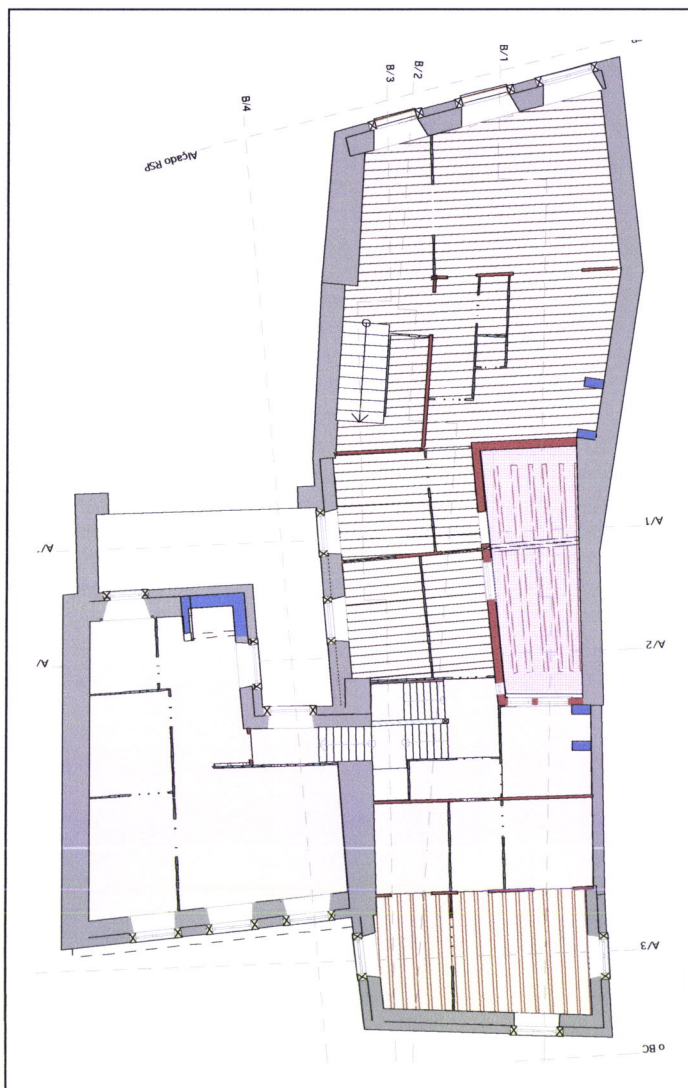
Planta Piso 1, Escala 1:200
