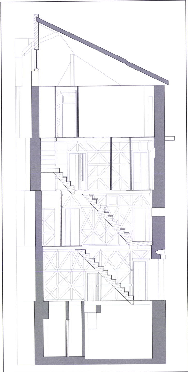
Corte 1, Escala 1:100
