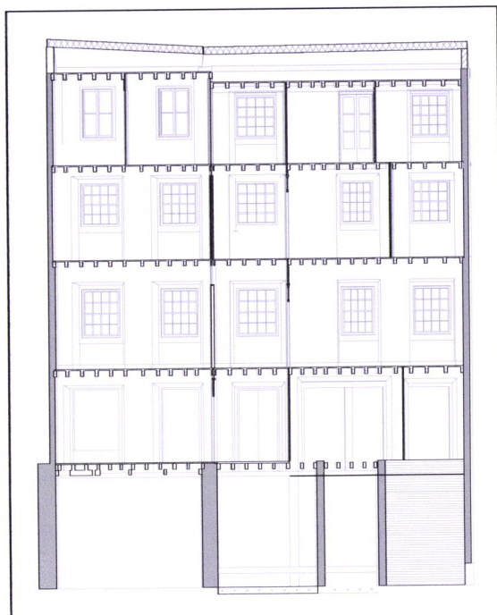
Corte A3, Escala 1:200
