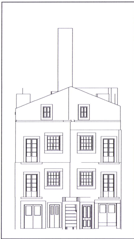
Alçado da Rua de São Pedro, Escala 1:200
