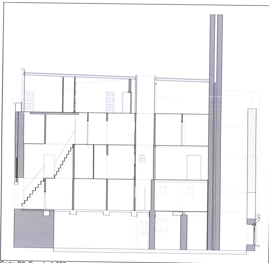
Corte B2, Escala 1:200
