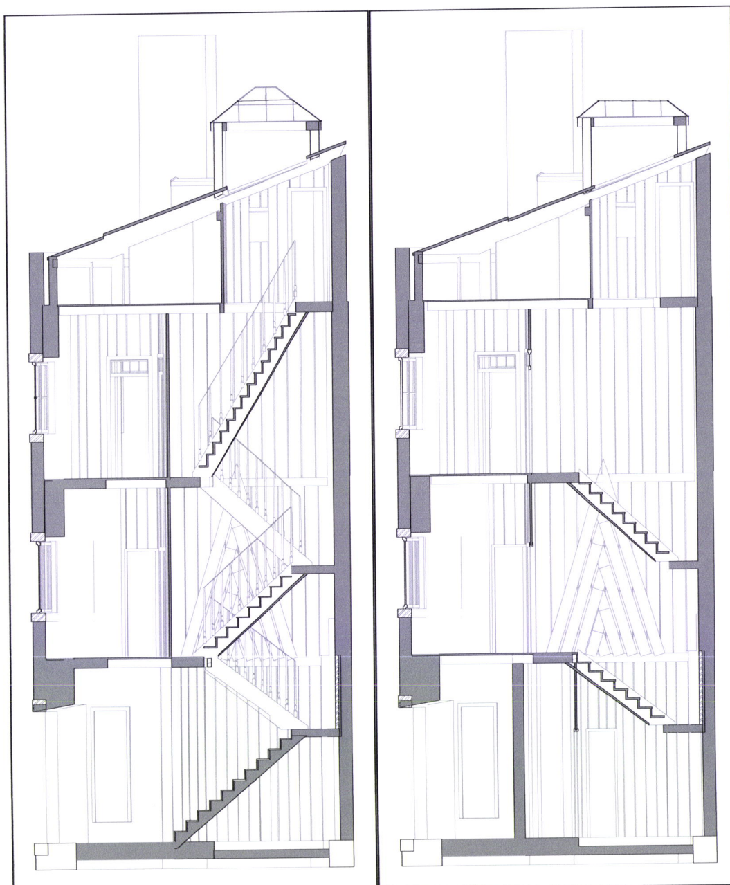
Cortes 1 e 3, Escala 1:100
