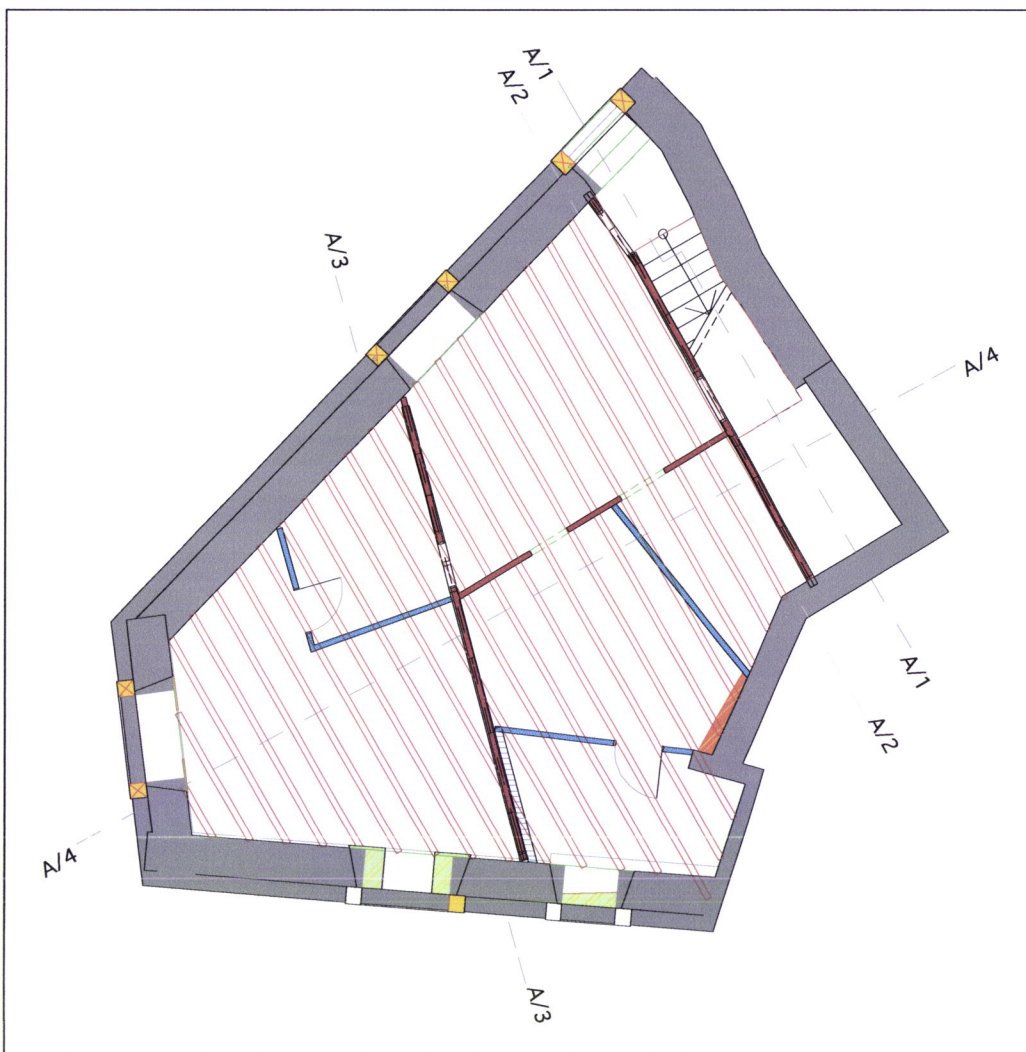
Planta Piso 1, Escala 1:100
