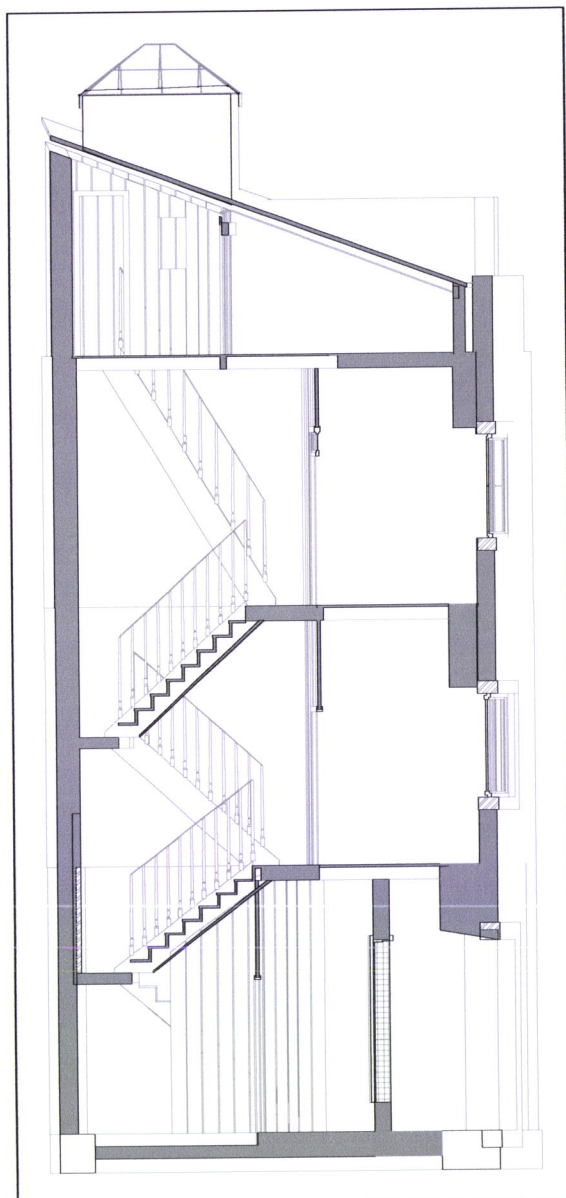
Corte 2, Escala 1:100
