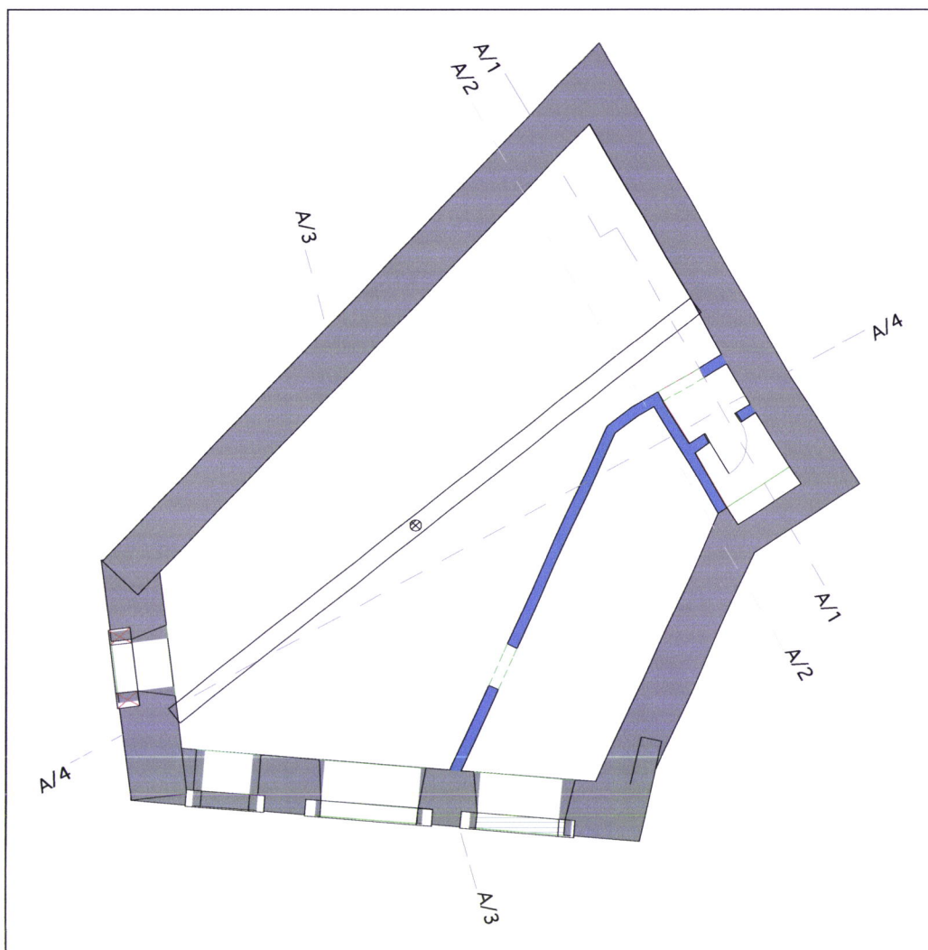
Planta Piso 0, Escala 1:100
