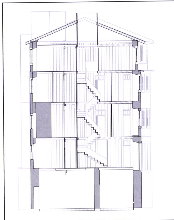
Corte B1, Escala 1:200
