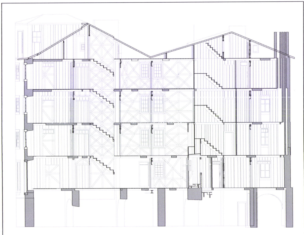
Corte B2, Escala 1:200
