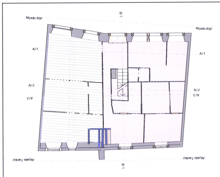
Planta Piso 0, Escala 1:200
