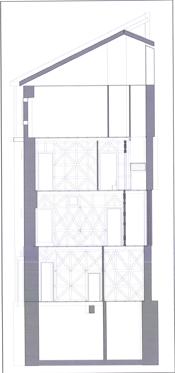
Corte 11, Escala 1:100
