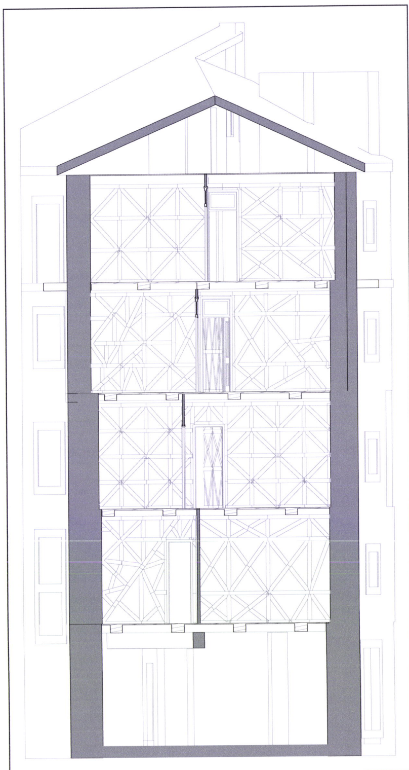
Corte 14, Escala 1:100
