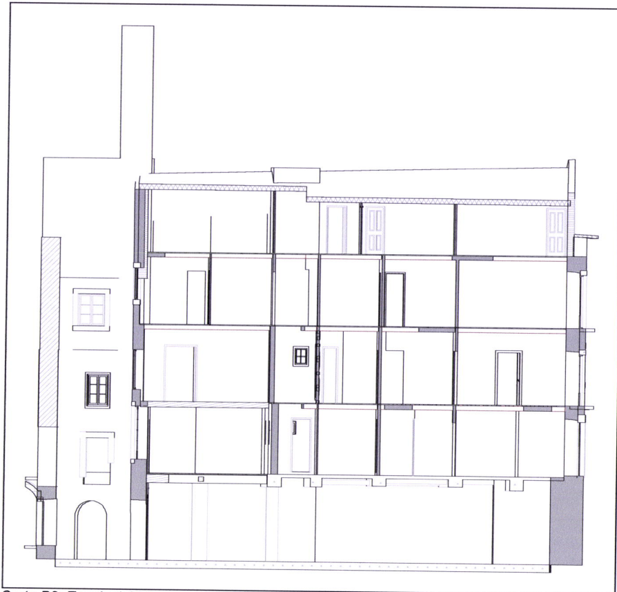
Corte B3, Escala 1:200
