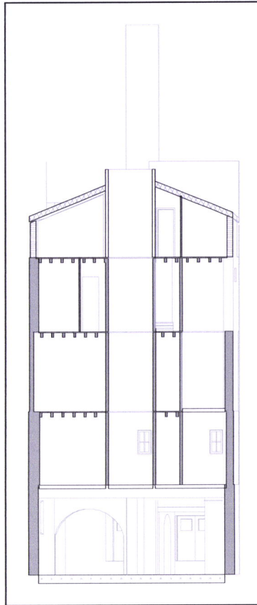
Corte A1, Escala 1:200
