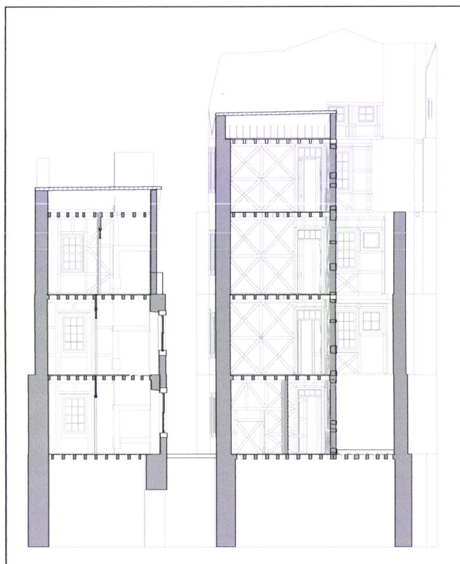
Corte A2, Escala 1:200
