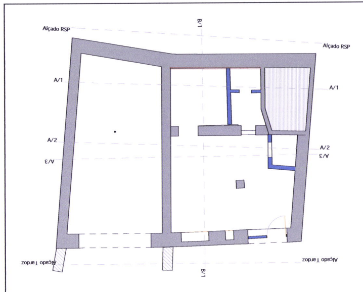
Planta Piso -1, Escala 1:200
