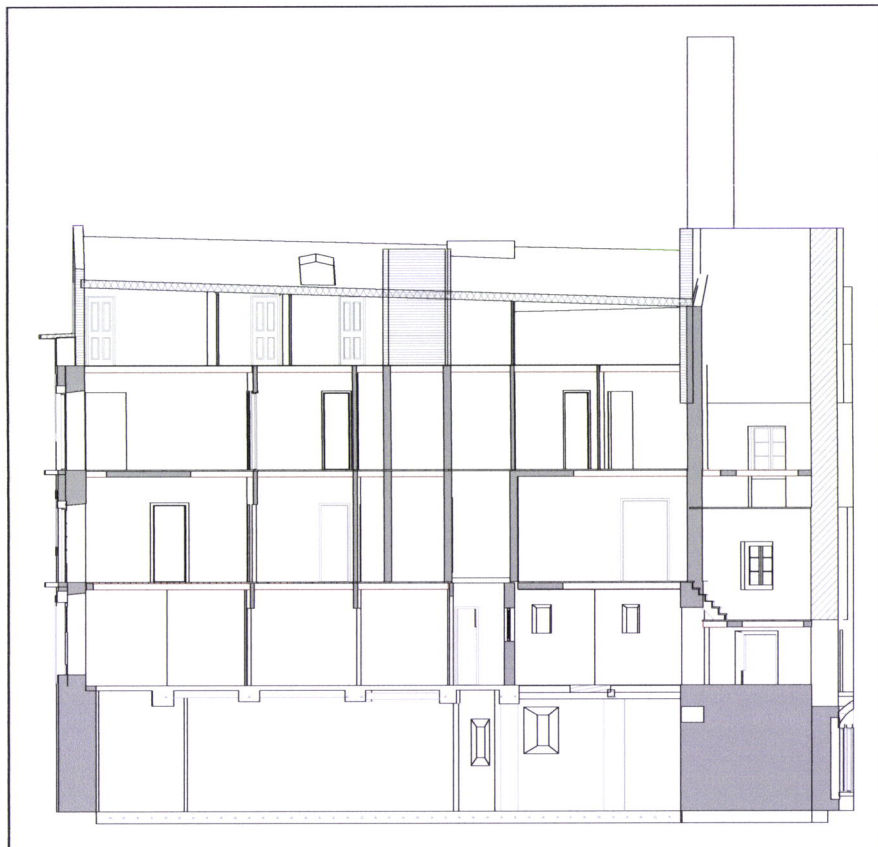
Corte B1, Escala 1:200
