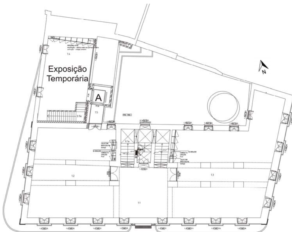
Planta do Museu Municipal de Portalegre (2012) - Piso 1
