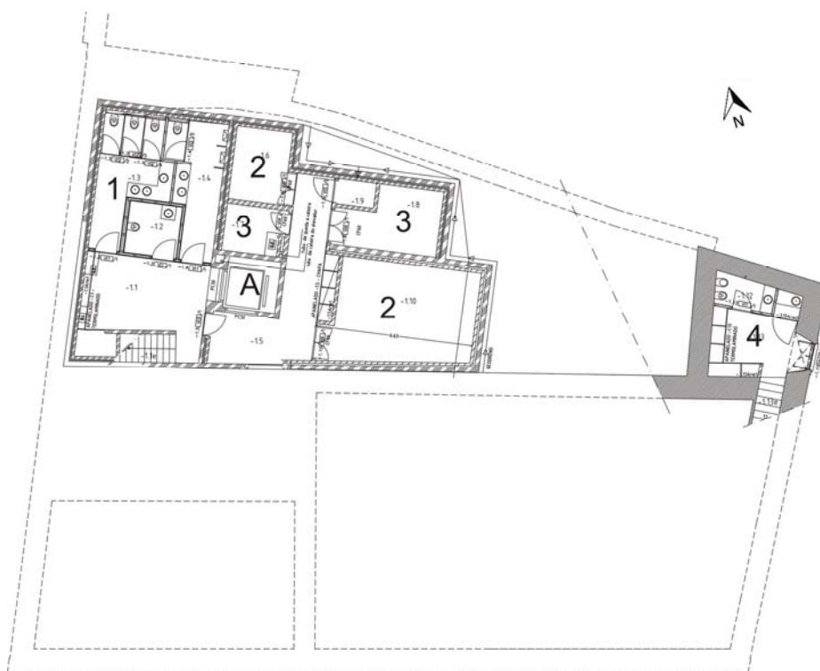
Planta do Museu Municipal de Portalegre (2012) - Piso - 2
