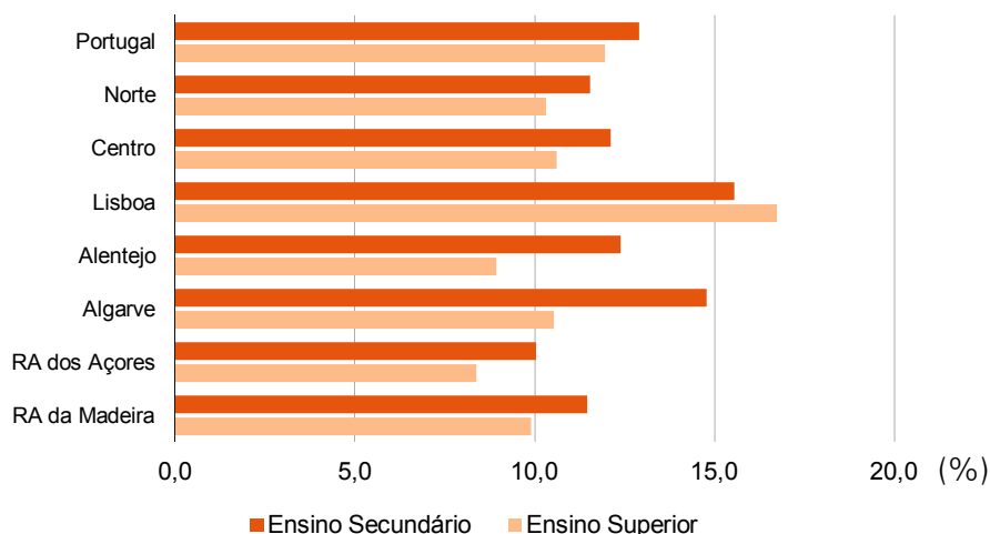
● Gráfico 1.4.3 População residente segundo o nível de ensino mais elevado e completo por NUTS II, em 2011
