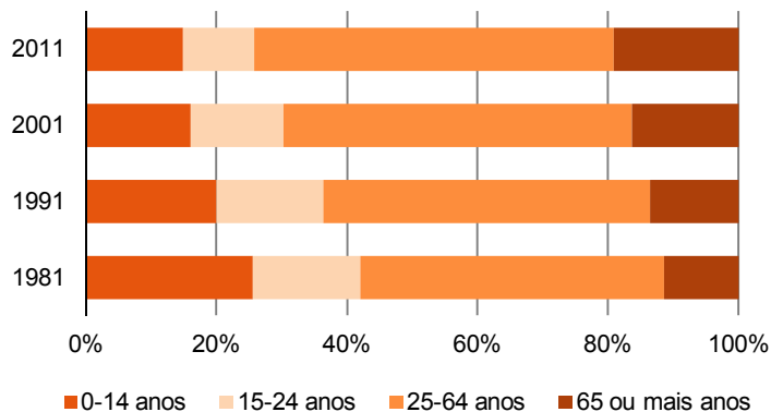
● Gráfico 1.2.1 Estrutura da população residente em Portugal por grupos etários em 1981, 1991, 2001, 2011
