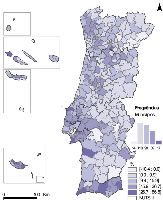
● Cartograma 3.1.1 Taxa de variação dos edifícios por município, 2001-2011
