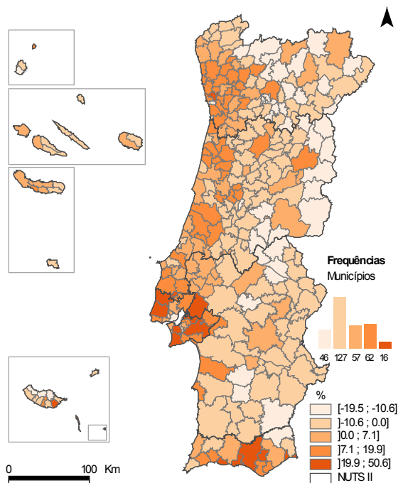
● Cartograma 1.1.1 Taxa de variação da população por município 1991-2001
