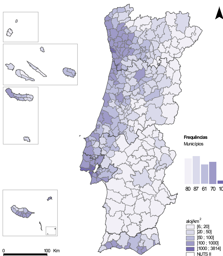
● Cartograma 3.1.3 Densidade de alojamentos por município, em 2011
