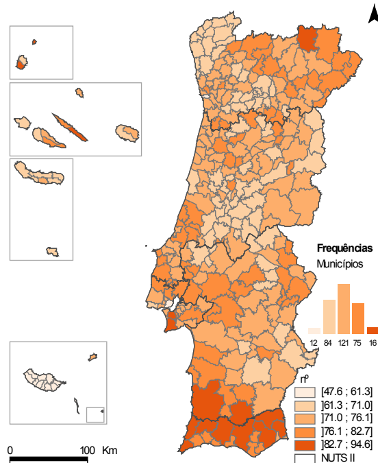
● Cartograma 1.2.2 Relação de masculinidade da população residente com 65 ou mais anos por município, 2011
