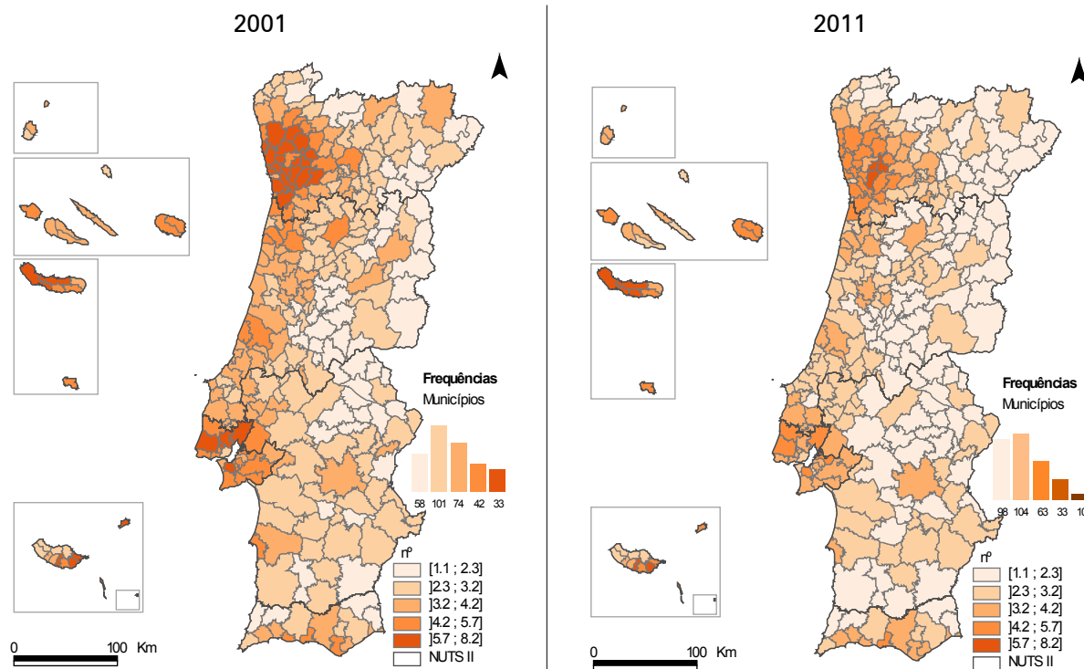
● Cartograma 1.2.4 Índice de sustentabilidade potencial por município
