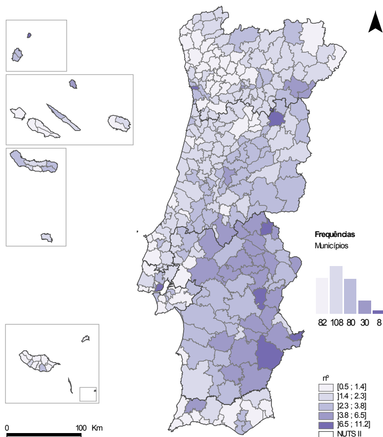
● Cartograma 3.2.2 Índice de envelhecimento dos edifícios por município, em 2011
