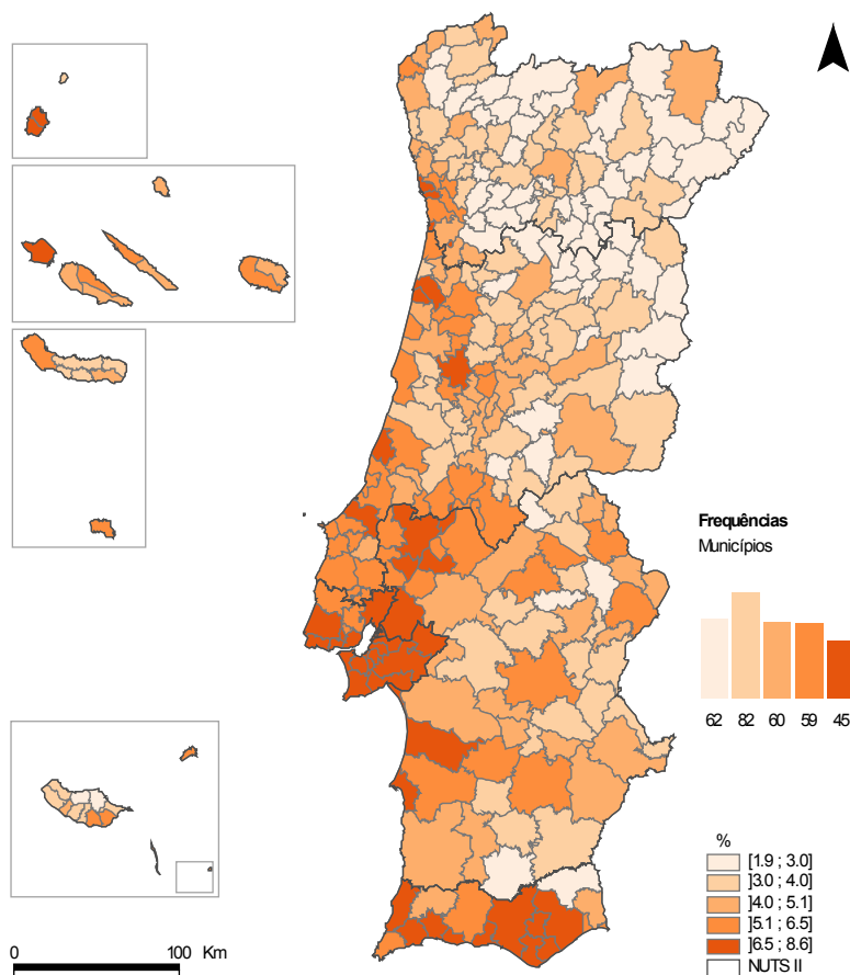
● Cartograma 1.3.1 Percentagem da população divorciada por município em 2011
