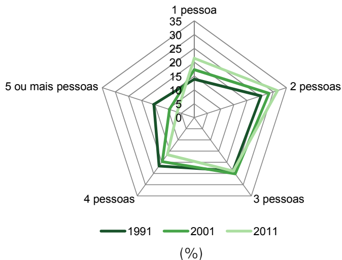
● Gráfico 2.2.1 Famílias clássicas segundo a dimensão, em 1991, 2001 e 2011
