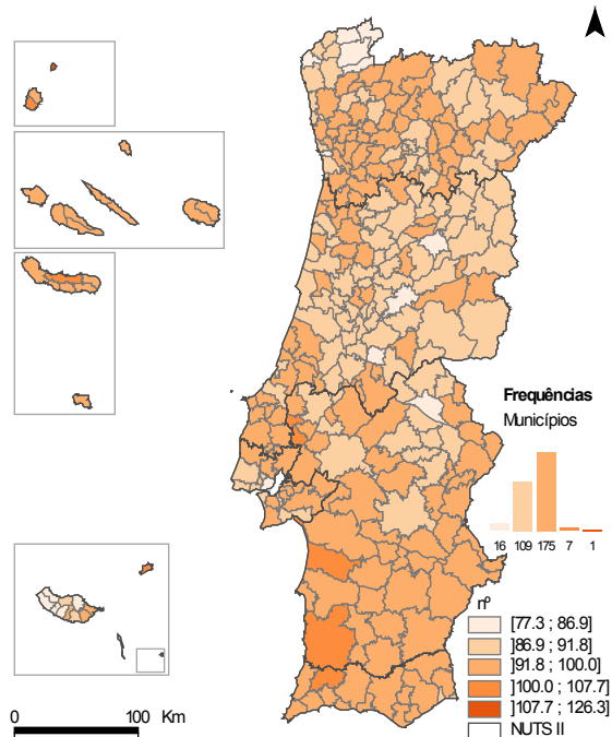
● Cartograma 1.2.1 Relação de masculinidade da população residente por município, 2011
