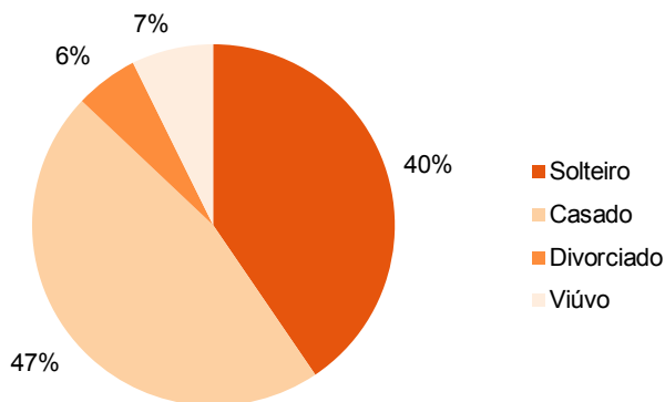
● Gráfico 1.3.1 Distribuição da população residente em Portugal segundo o estado civil em 2011
