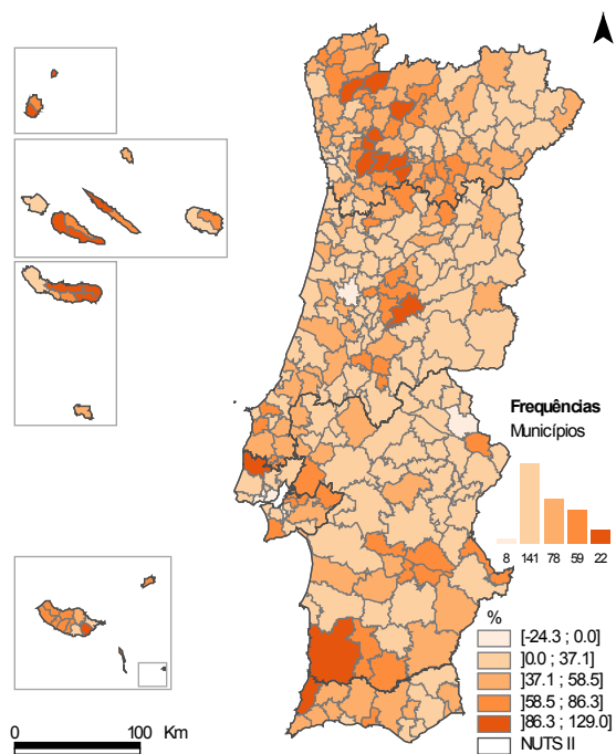
● Cartograma 1.4.1 Variação da população residente com ensino secundário completo por município, 2001-2011
