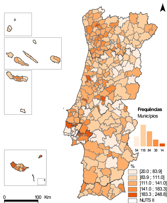
● Cartograma 1.4.2 Variação da população residente com ensino superior completo por município, 2001-2011
