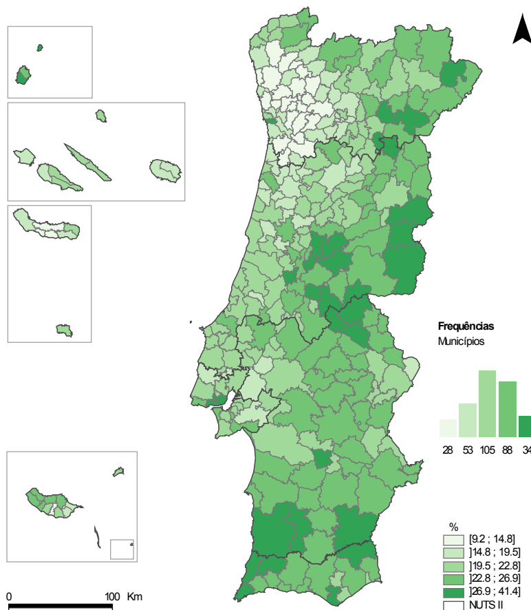
● Cartograma 2.2.2 Percentagem de famílias unipessoais por município, em 2011
