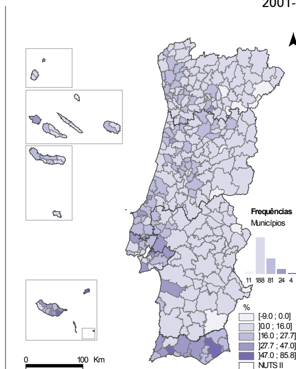
● Cartograma 3.1.2 Taxa de variação dos alojamentos por município, 2001-2011
