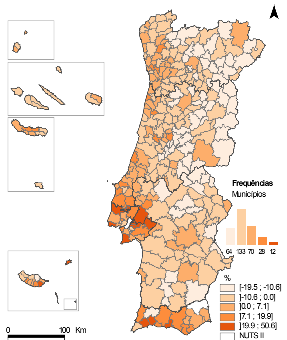
● Cartograma 1.1.2 Taxa de variação da população por município 2001-2011
