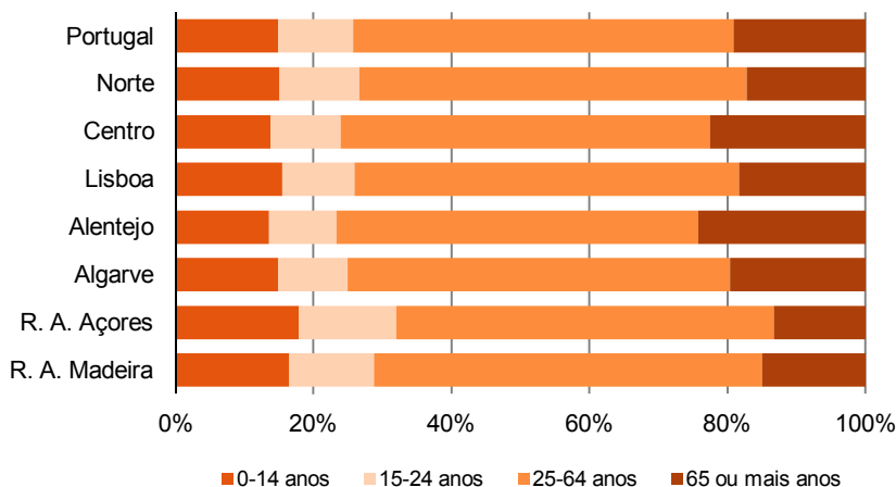
● Gráfico 1.2.2 Estrutura da população residente por grupos etários por NUTS II em 2011
