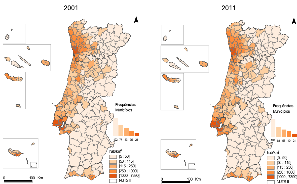
● Cartograma 1.1.3 Densidade populacional por município
