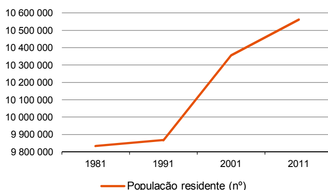
● Gráfico 1.1.1 Evolução da população residente em Portugal, 1981-2011
