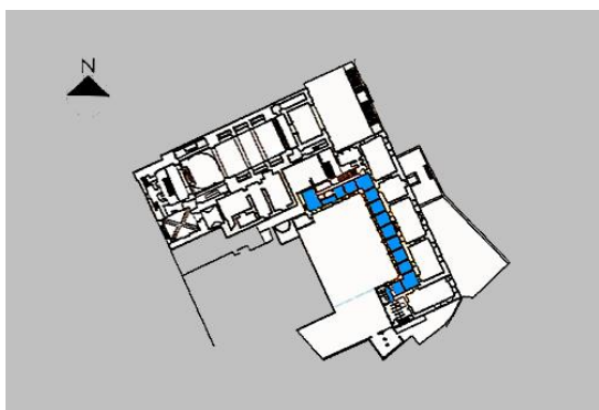
Fig. 12 – Convento de Nossa Senhora do Carmo. Planta do conjunto.
