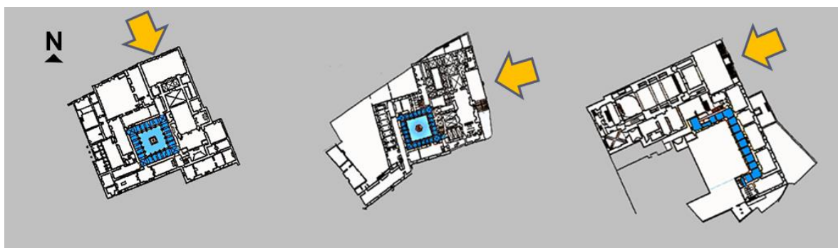
Fig. 83 – Plantas dos conventos carmelitas de Évora.
