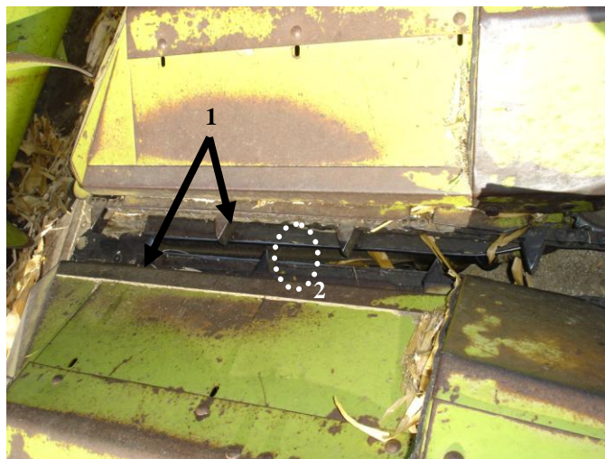
Vista superior do mecanismo de colheita de uma linha de milho: 1 – Correntes transportadoras; 2 – Folga entre chapas que deixa passar os caules mas não as espigas (arrancando-as).
