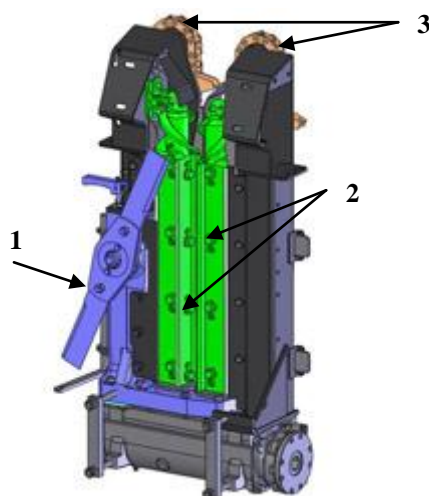
Vista inferior do mecanismo de colheita de uma linha de milho: 1 – rotor de facas para ceifar os caules; 2- rolos para entalar e puxar os caules na direcção do solo; 3 – Correntes transportadoras.
