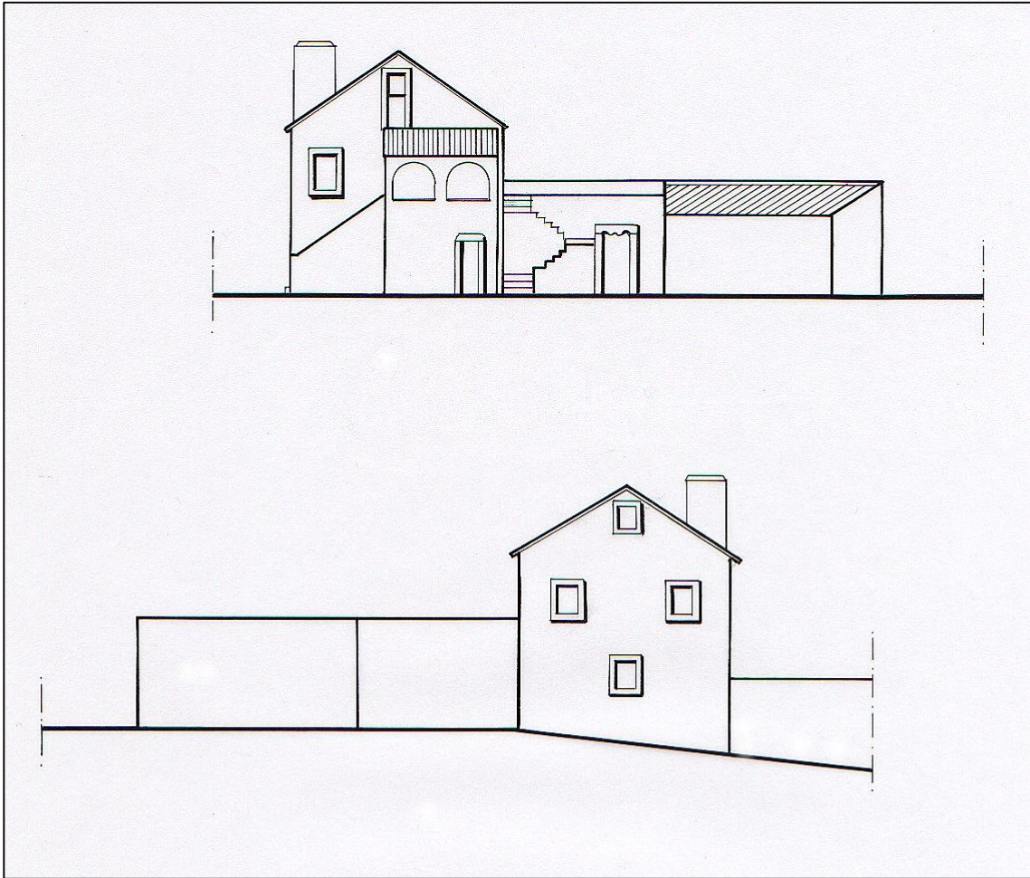
Fig. 13 – Turquel. Quinta da Granja, alçado sul. Esc.1/200
