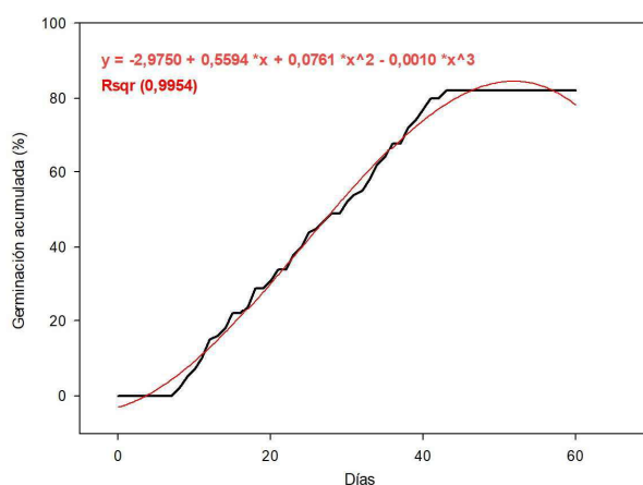
Figura 19. Distribución de la curva de germinación de las semillas de Quercus canariensis Willd., a lo largo del año 2018-2019, en las condiciones de oscuridad y temperatura previamente indicadas, con una humedad por encima del 80%. En rojo la curva de tendencia con R^2 , que nos ofrece el ajuste de los datos observados a una curva de tipo polinomial grado 3.
