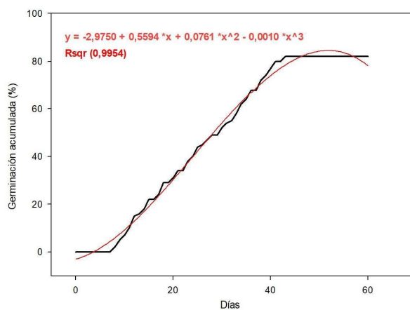
Figura 19. Distribuição da curva de germinação das sementes de Quercus canariensis Willd., ao longo do ano 2018–2019, nas condições de escuridão e temperatura indicadas anteriormente, com humidade acima de 80%. A vermelho a curva de tendência com R^2 , que nos oferece o ajuste dos dados observados para uma curva polinomial do tipo 3 graus.
