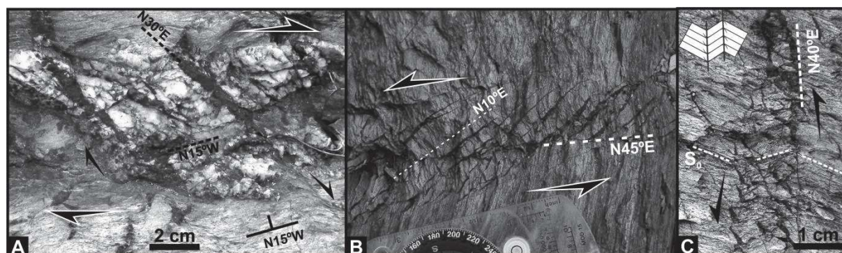
FIGURA 1 – Estruturas menores sinérgicas com a mineralização: (A) veio de quartzo, cortado por veios de óxidos, desenvolvido paralelamente a S_0 ; (B) veios en-echelon compatíveis com cinemática esquerda segundo uma direcção N45^\circ E ; (C) banda kink N40^\circ E esquerda com abertura de veios sin-cinemáticos.
