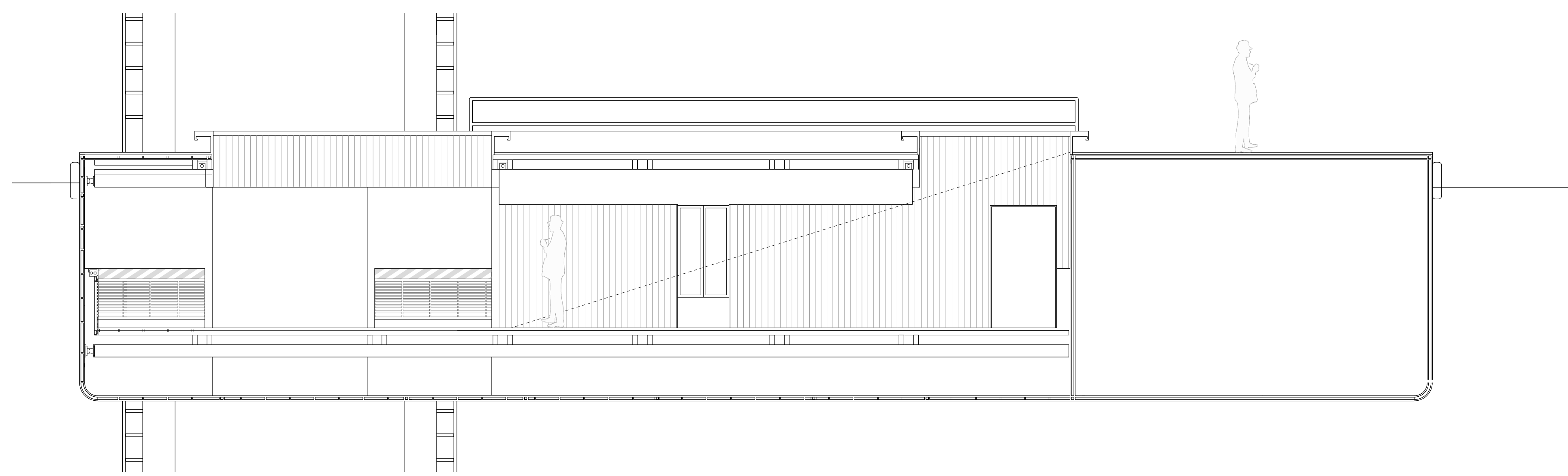
secção transversal EE'1 do volume submerso . 1:50
