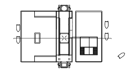
EXPLORAÇÃO AQUÍCOLA E4 Corte transversal EE' 1:100
