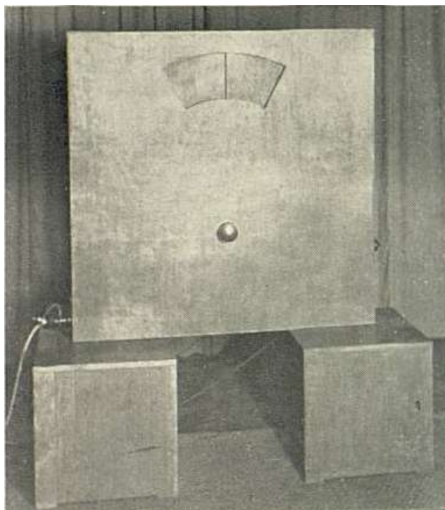
Figura 4.7 – Tradutor de configurações sonoras em configurações luminosas
