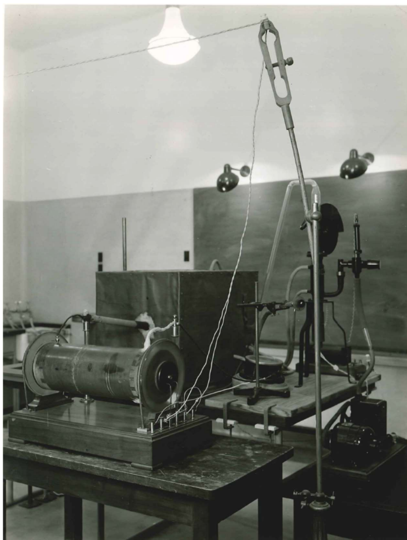
Figura 4.3 – Instalação para espectrografia de raios X
