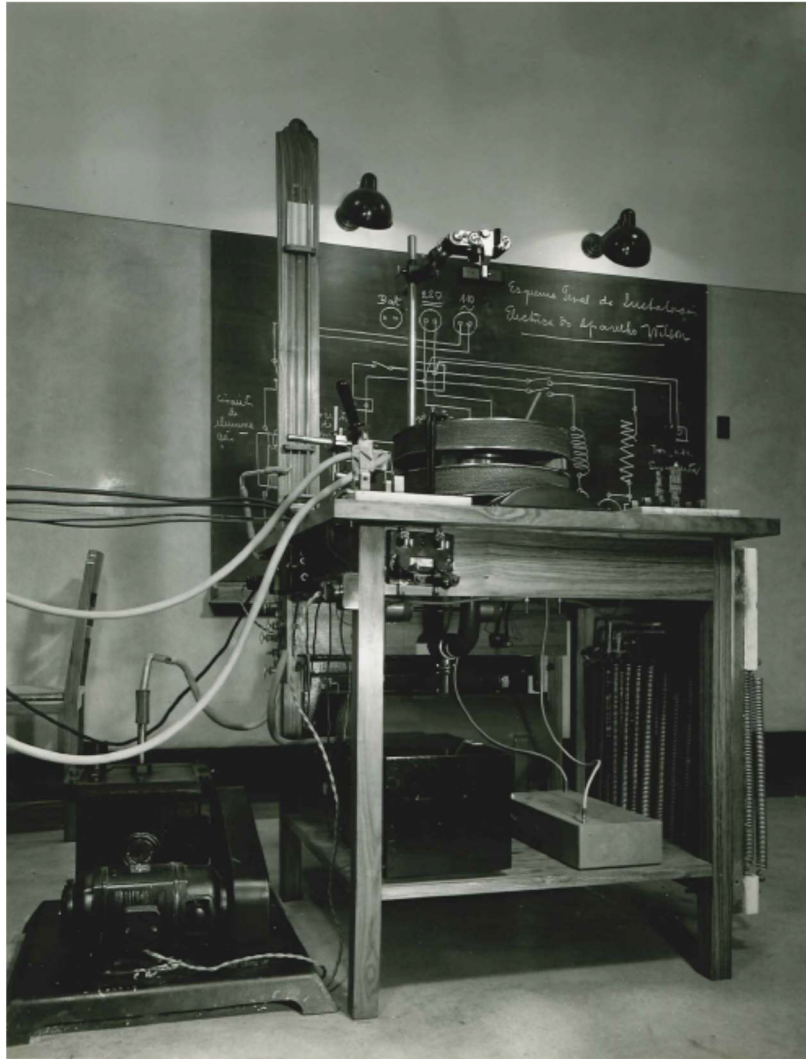
Figura 4.4 – Câmara de Wilson
