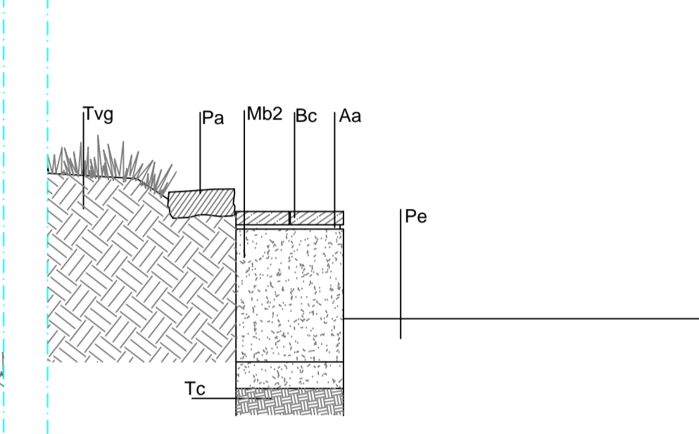
Pormenor 5 - Esc:1/20
