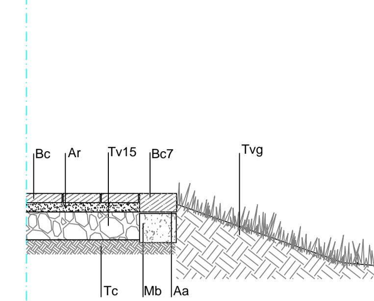
Pormenor 2 - Esc:1/20
