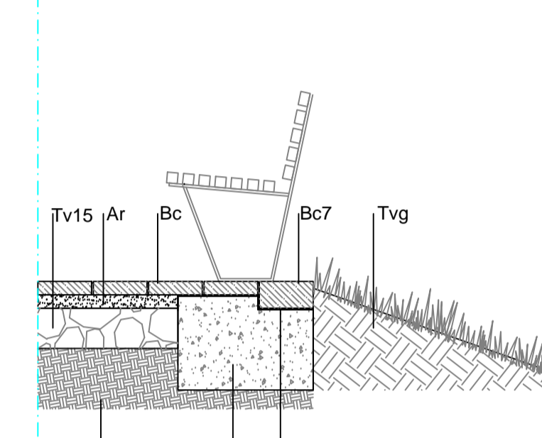
Pormenor 4 - Esc:1/20
