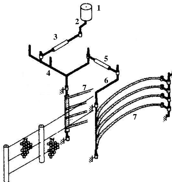
Fig. 1.7 – Cadeia cinemática dos sacudidores
