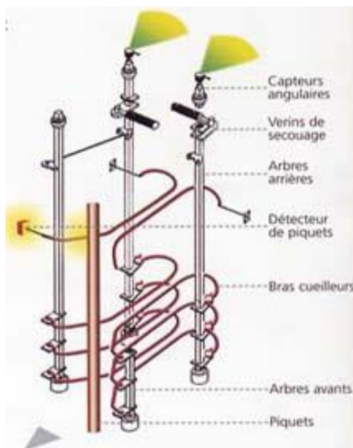
Fig. 1.43 http://www.pellenc.com/
