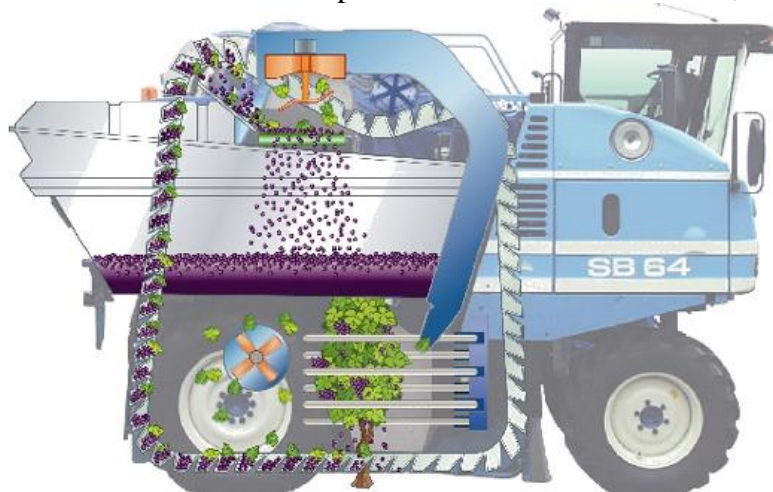
Fig. 1.19 – Máquina Braud New Holland
