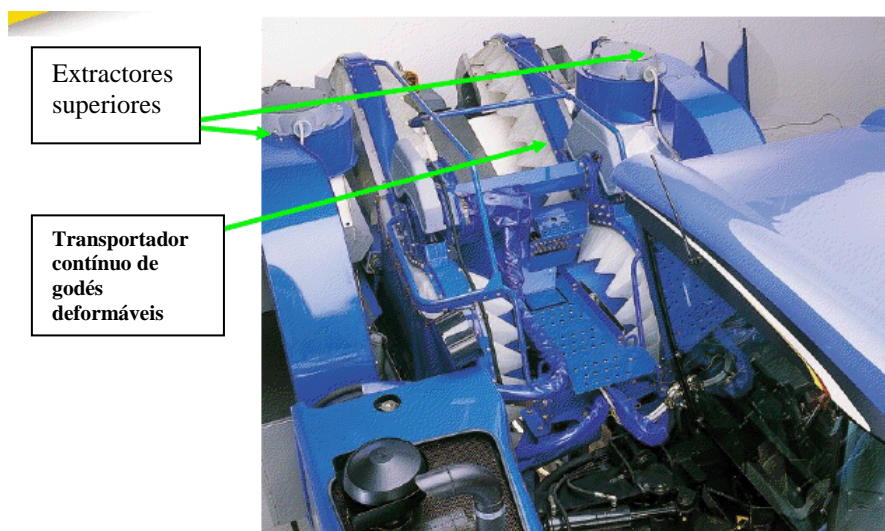
Fig. 1.25 – Extractor de limpeza superior de uma máquina Braud New Holland
