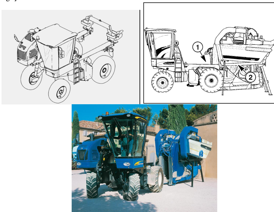
Fig. 1.1 – Unidade tractor e unidade de colheita http://www.newholland.com/
