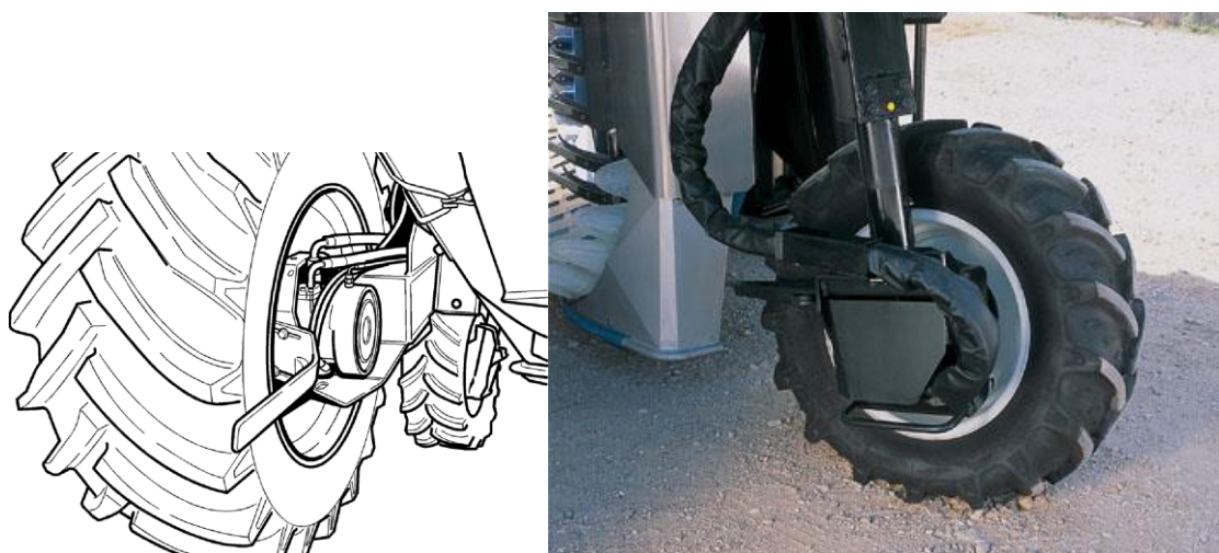
Fig. 1.2 – motor hidráulico nas rodas http://www.newholland.com/
