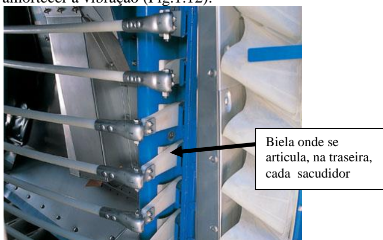
Fig. 1.12 – Articulação dos sacudidores http://www.newholland.com/
