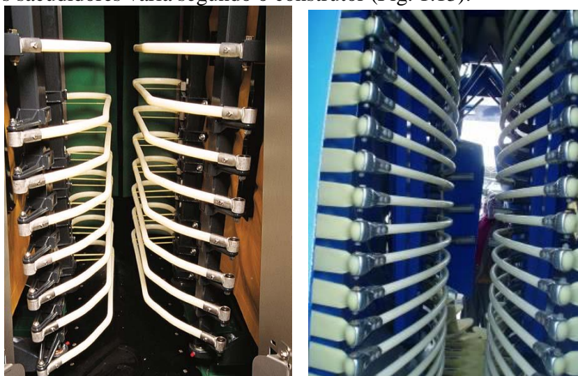
Fig. 1.13 - sacudidores http://www.pellenc.com/ (esquerda); Máquina Braud New Holland Modelo VX7090 na Expoliva 2009 – Jaen - Espanha
