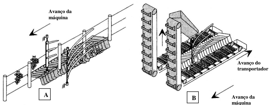
Fig. 1.17 – (A) Princípio de funcionamento das escamas retráteis ; (B) Esquema dos tapetes transportadores para o sistema de armazenamento
