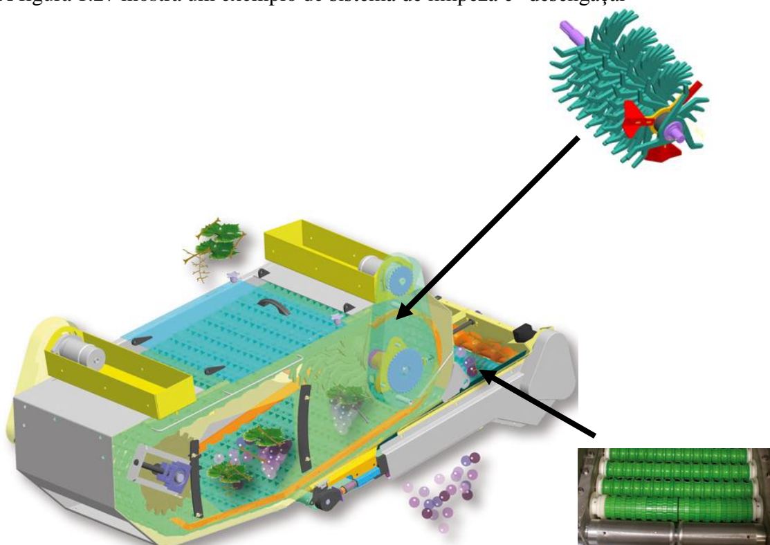
Fig. 1.27 – Sistema de limpeza e para desengaçar http://www.gregoire.fr
