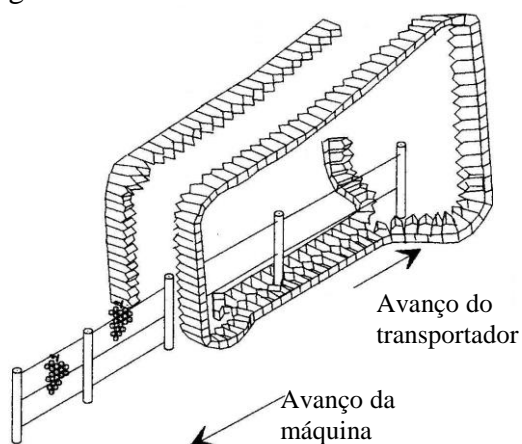
Fig.1.18 - Transportador contínuo de godés deformáveis (G. Vromandt)
