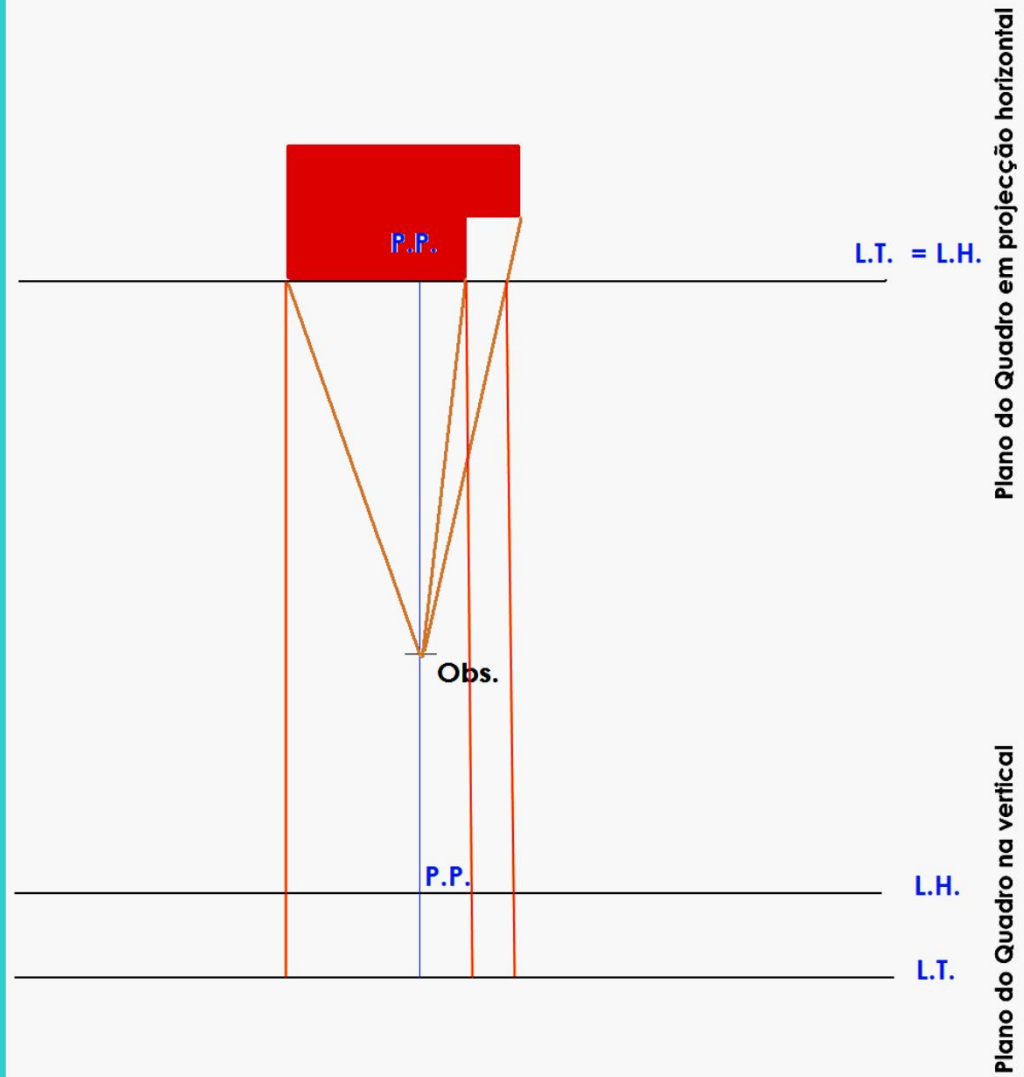
Perspectiva Central
