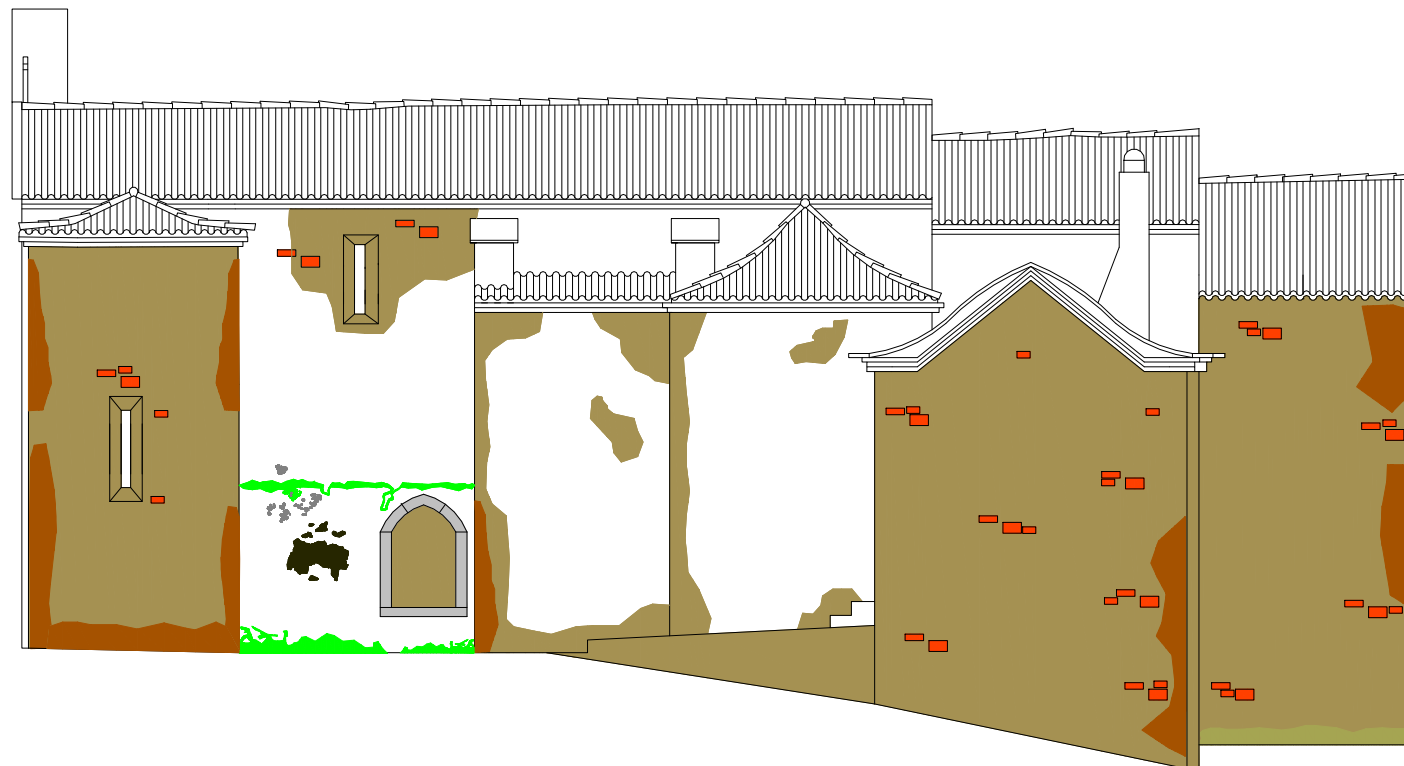
Alçado Sul
