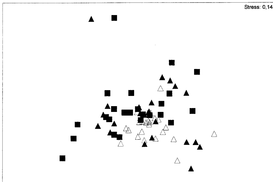
Figura 4.16- Ordenação bidimensional por MDS não métrica das 72 réplicas amostradas numa experiência manipulativa de remoção de lapas realizada no nível inferior de maré de duas praias do litoral rochoso alentejano, segundo o delineamento apresentado na tabela 4.3 e com base nos valores de variação percentual, entre os dois períodos considerados, da área de rocha nua e da área primariamente coberta por algas encrustantes moles, algas encrustantes duras e cracas, estimados em territórios alimentares de lapas: controlo ( \triangle ); remoção de lapas de tamanho grande ( \blacktriangle ); remoção de todas as lapas ( \blacksquare ). A matriz de similaridade foi calculada com o coeficiente de Bray-Curtis, após transformação por raiz quadrada.
