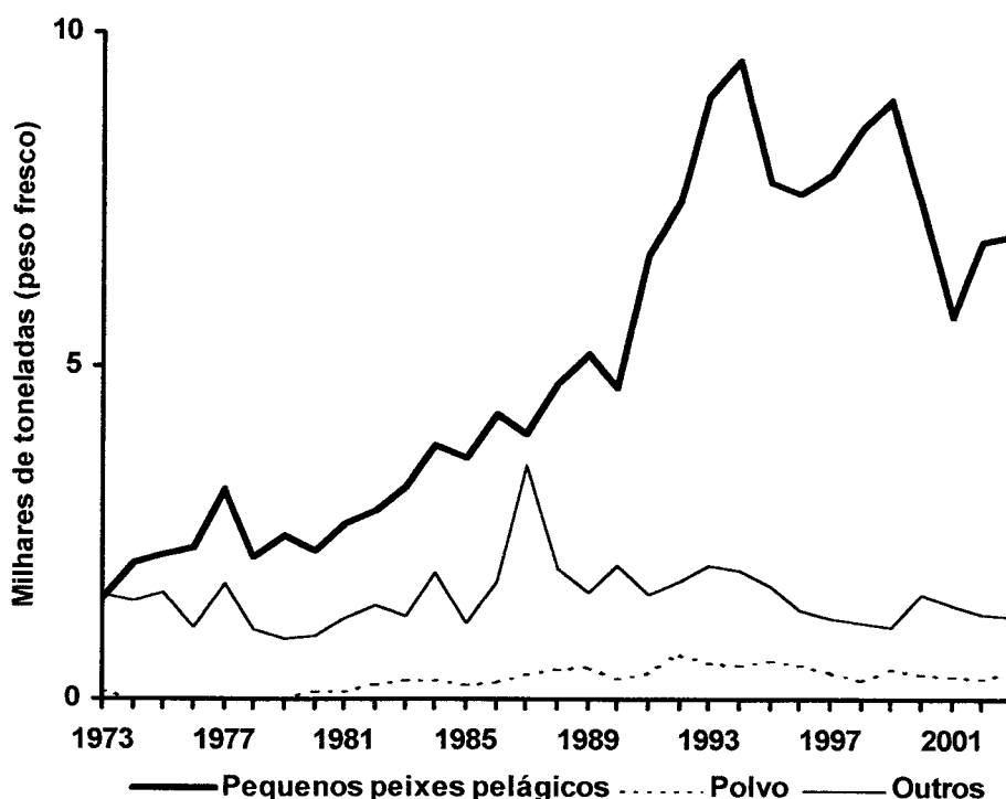
Figura 7.3- Peso do pescado marinho desembarcado em lotas do Alentejo - variação anual entre 1973 e 2003 (com base em estatísticas de pesca publicadas pelo Instituto Nacional de Estatística entre 1973 e 2003, inclusive; INE e DGPA, 1998). "Pequenos peixes pelágicos" são: biqueirão, carapaus (incluindo chicharro), cavala, sarda e sardinha. "Outros" corresponde a outros peixes marinhos, crustáceos e outros moluscos.
