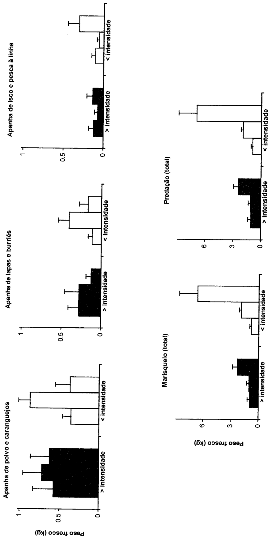
Figura 3.1- Variação do peso (média+erro padrão) do pescado capturado por pescador em diversas actividades de predação no litoral rochoso alentejano, no final de períodos de baixa-mar de marés vivas do Verão de 1999, segundo o delineamento da questão 3.1A: praias sujeitas a maior (barras pretas) intensidade de exploração são, da esquerda para a direita, Amoreiras/Casca/Oliveirinha, Burrinho/Porto Covo/Queimado e Almogrove; praias sujeitas a menor (barras brancas) intensidade de exploração são, da esquerda para a direita, Caniceira, Nascedios e Cabo Sardão; 22 réplicas. Alguns eixos de ordenadas possuem escalas diferentes.
