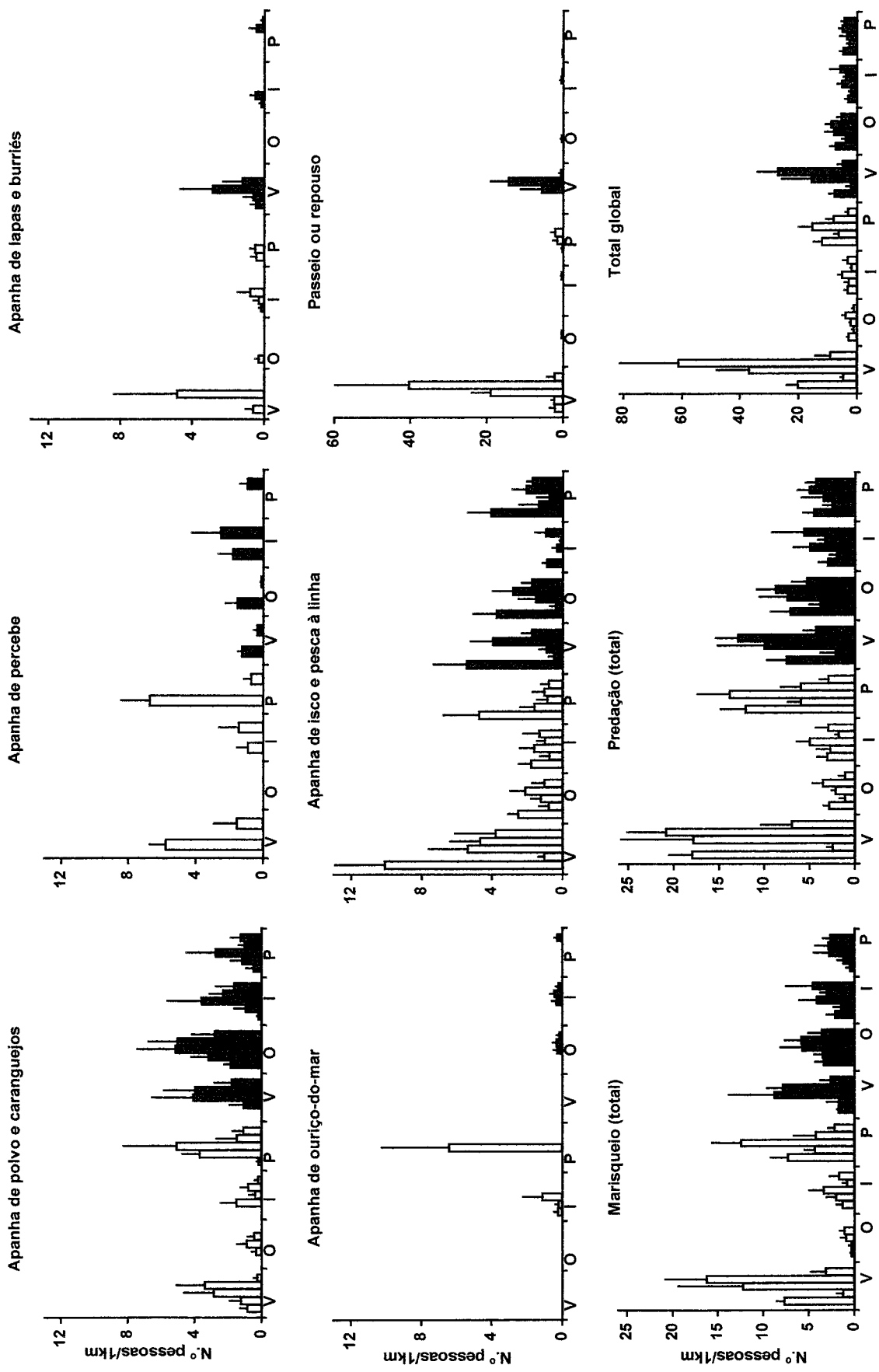
Figura 2.2- Variação da abundância (média+erro padrão) de pessoas em diversas actividades de utilização do litoral rochoso alentejano, em baixa-mar de águas vivas e dias úteis, segundo o delineamento da questão 2.1A (tabela 2.3): barras brancas=1994/5; barras pretas=1995/6; V=Verão; O=Outono; P=Primavera; da esquerda para a direita, Cabo de Sines, Vale Marim, Amoreiras/Casca/Oliveirinha, Almogrove e Cabo Sardão, e, no caso da apanha de percebe, Cabo de Sines, Almogrove e Cabo Sardão; 6 réplicas (3 locais por praia x 2 datas por estação do ano). Alguns eixos de ordenadas possuem escalas diferentes.
