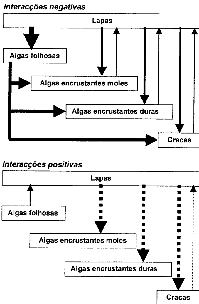
Figura 4.17- Direcção e intensidade relativa de interações negativas e positivas sugeridas pelos resultados de uma experiência manipulativa de remoção de lapas efectuada num nível inferior de maré do litoral rochoso alentejano (ver texto). Linhas contínuas: efeitos directos; linhas descontínuas: efeitos indirectos. A largura das linhas está directamente relacionada com a intensidade dos efeitos.
