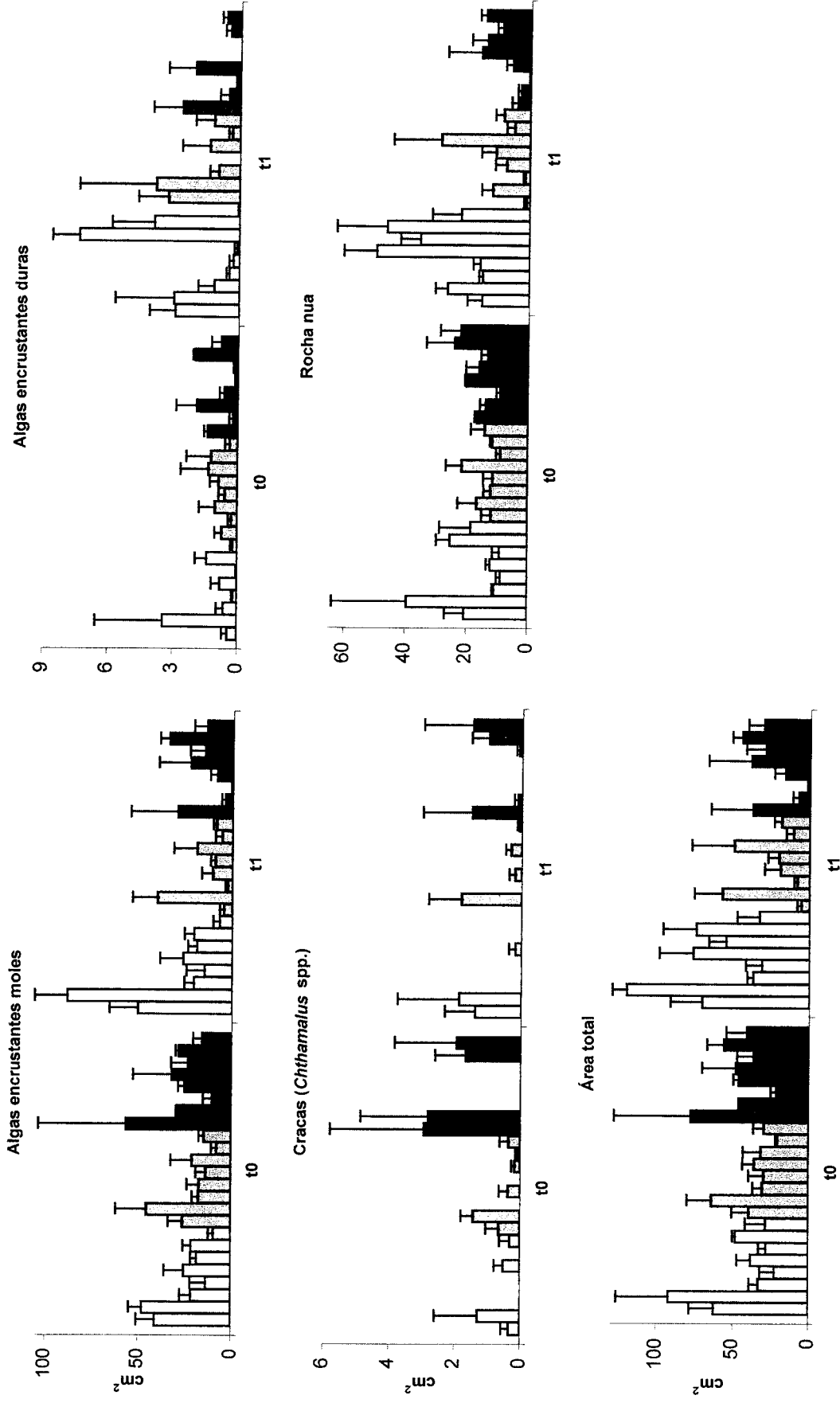
Figura 4.13- Variação da área (média+erro padrão) primariamente coberta por algas encrustantes moles, algas encrustantes duras, cracas ( Chthamalus spp.) e rocha nua (não coberta por macrobentos ou ocupada por lapas) em territórios alimentares de lapas, e da área total dos mesmos territórios, no âmbito de uma experiência manipulativa de remoção de lapas efectuada no nível inferior de maré de duas praias do litoral rochoso alentejano (Oliveirinha/Burrinho - praia 1; Nascedios - praia 2), segundo o delineamento apresentado na tabela 4.3: não remoção de lapas (barras brancas), remoção de lapas de tamanho grande, com 30mm ou mais de comprimento máximo da concha (barras cinzentas), e remoção de todas as lapas (barras pretas); da esquerda para a direita, área 1/local 1/praias 1, área 2/local 1/praias 1, ..., área 2/local 2/praias 2; amostragem efectuada no início da experiência (t0 - Setembro/Outubro de 1997) e seis a nove meses depois (t1 - Março/Junho de 1998); 3 réplicas. Os eixos de ordenadas possuem escalas diferentes.
