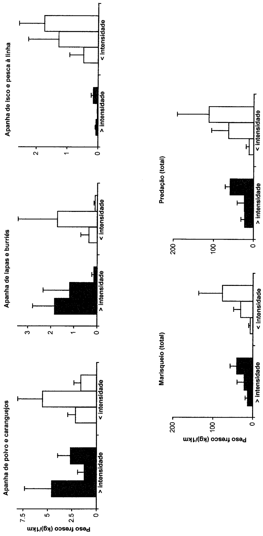
Figura 3.5. Variação do peso (média+erro padrão) do pescado capturado pela totalidade dos pescadores observados em diversas actividades de predação no litoral rochoso alentejano, no final de períodos de baixa-mar de marés vivas do Verão de 1999, segundo o delineamento da questão 3.2C: praias sujeitas a maior (barras pretas) intensidade de exploração são, da esquerda para a direita, Amoreiras/Casca/Oliveirinha, Burrinho/Porto Covo/Queimado e Almogrove; praias sujeitas a menor (barras brancas) intensidade de exploração são, da esquerda para a direita, Caniceira, Nascedios e Cabo Sardão; 3 réplicas (cada réplica é o produto do peso médio de pescado obtido por pescador e do número total de pescadores observados em actividade). Alguns eixos de ordenadas possuem escalas diferentes.
