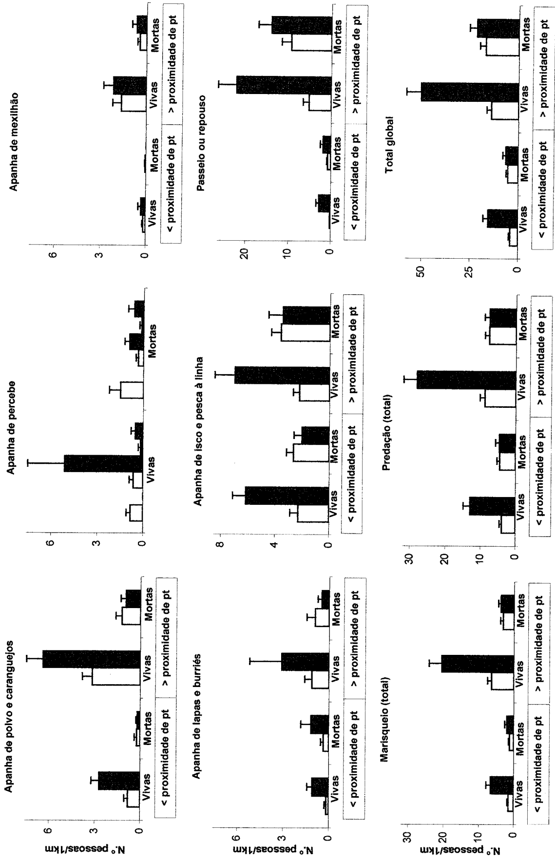
Figura 2.6- Variação da abundância (média+erro padrão) de pessoas em diversas actividades de utilização do litoral rochoso alentejano, em baixa-mar e no Verão de 1995, segundo o delimitamento da questão 2.2C (tabela 2.4): barras brancas=dias úteis; barras pretas=dias não úteis; Vivas=marés vivas; Mortas=marés mortas; pt=praias arenosas turísticas; praias com < proximidade de pt são Cabo de Sines, Vale Marim, Nascedios e Cabo Sardão; praias com > proximidade de pt são Amoreiras/Casca/Oliveirinha, Burrinho/Porto Covo, Caniceira/Queimado, e Almogrove; 36 réplicas (4 praias x 3 locais por praia x 3 datas por estação do ano); no caso da apanha de percebe, as praias são, da esquerda para a direita, Cabo de Sines, Almogrove e Cabo Sardão, e o número de réplicas é 9 (3 locais por praia x 3 datas por estação do ano). Alguns eixos de ordenadas possuem escalas diferentes.
