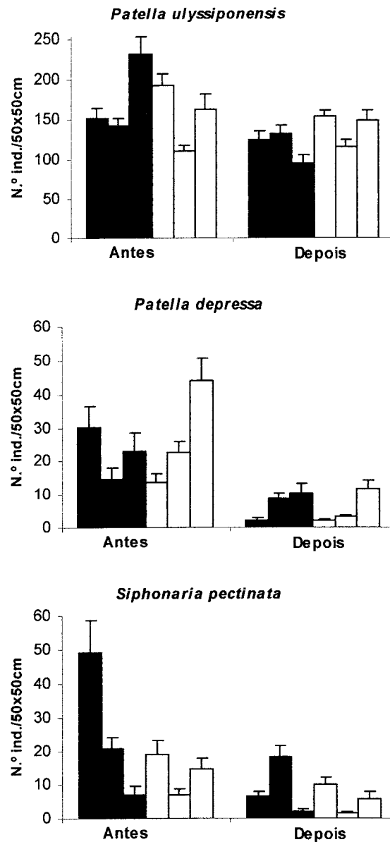
Figura 4.2- Variação da densidade (média+erro padrão) total das espécies de lapas mais abundantes no nível inferior de maré de diversas praias do litoral rochoso alentejano sujeitas a diferente intensidade de exploração humana, segundo o delineamento apresentado na tabela 4.1: praias sujeitas a maior (barras pretas) intensidade de exploração são, da esquerda para a direita, Oliveirinha, Burrinho e Almogrove; praias sujeitas a menor (barras brancas) intensidade de exploração são, da esquerda para a direita, Caniceira, Nascedios e Cabo Sardão; amostragem efectuada antes (Antes) e depois (Depois) do Verão de 1999; 32 réplicas (2 datas por período do ano x 2 locais por praia x 8 réplicas por local). Alguns eixos de ordenadas possuem escalas diferentes.
