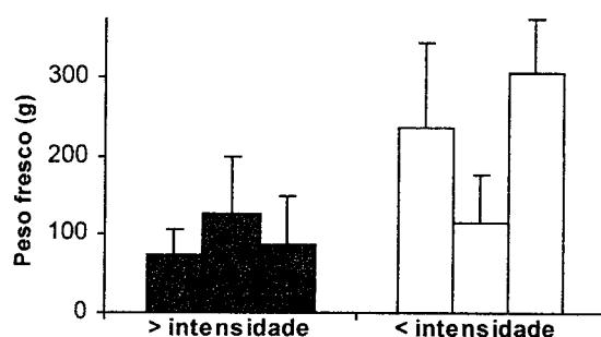
Figura 3.7- Variação do peso (média+erro padrão) do pescado capturado por pescador em trinta minutos de actividade de pesca à linha no litoral rochoso alentejano, em períodos de enchente do Verão de 1999, segundo o delineamento da questão 3.3A: praias sujeitas a maior (barras pretas) intensidade de exploração são, da esquerda para a direita, Amoreiras/Casca/Oliveirinha, Burrinho/Porto Covo/Queimado e Almogrove; praias sujeitas a menor (barras brancas) intensidade de exploração são, da esquerda para a direita, Caniceira, Nascédios e Cabo Sardão; 10 réplicas. Alguns eixos de ordenadas possuem escalas diferentes.
