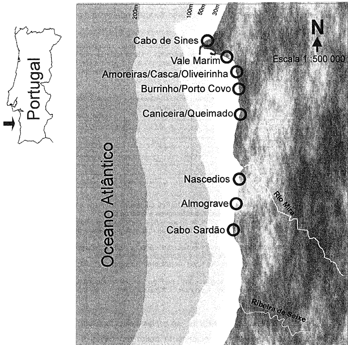
Figura 2.1- Localização das praias de amostragem utilizadas no estudo dos padrões de variação espacial e temporal da abundância de pessoas utilizando o litoral rochoso alentejano.
