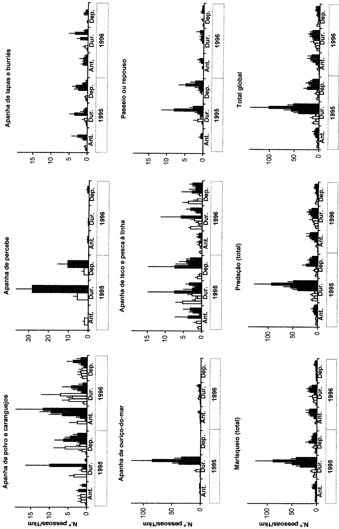
Figura 2.10. Variação da abundância (média+erro padrão) de pessoas em diversas actividades de utilização do litoral rochoso alentejano, em baixa-mar de marés vivas e nos períodos antes (Ant.), durante (Dur.) e depois (Dep.) da Páscoa de 1995 e 1996, segundo o delimitamento da questão 2.3C (tabela 2.5): barras brancas=dias úteis; barras pretas=dias não úteis; as praias amostradas são, da esquerda para a direita, Cabo de Sines, Vale Marim, Amoreiras/Casca/Oliveirinha e Burrinho/Porto Covo; no caso da apanha de percebe, a praia amostrada é Cabo de Sines; 6 réplicas (3 locais por praia x 2 datas por período). Alguns eixos de ordenadas possuem escalas diferentes.
