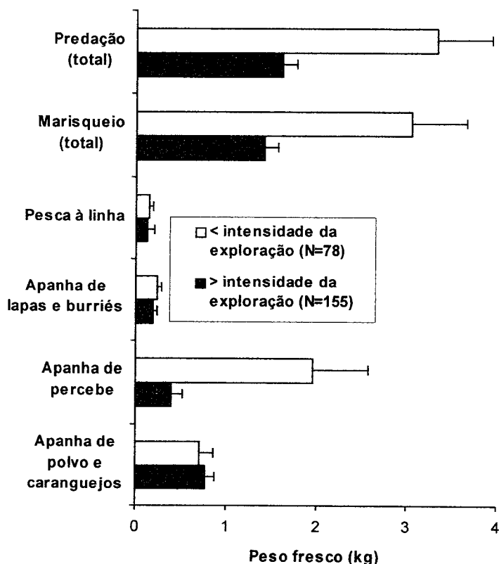
Figura 3.6- Variação do peso (média+erro padrão) do pescado capturado por pescador em diversas actividades de predação do litoral rochoso alentejano, considerando a totalidade das observações efectuadas no final de períodos de baixa-mar de marés vivas do Verão de 1999, em praias sujeitas a diferente intensidade de exploração, segundo o delineamento e as técnicas de amostragem referidas na secção 3.2; N- número total de réplicas (para além das 226 réplicas referidas na secção 3.2, foram também consideradas 7 observações efectuadas nos mesmos conjuntos de praias e períodos de amostragem).
