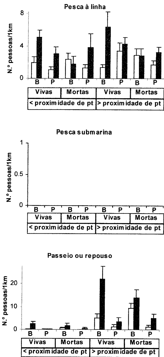
Figura 2.7- Variação da abundância (média+erro padrão) de pessoas em diversas actividades de utilização do litoral rochoso alentejano, no Verão de 1995, segundo o delineamento da questão 2.2D (tabela 2.4): barras brancas=dias úteis; barras pretas=dias não úteis; B=baixa-mar; P=preia-mar; Vivas=marés vivas; Mortas=marés mortas; pt=praias arenosas turísticas; praias com < proximidade de pt são Cabo de Sines, Vale Marim, Nascedios e Cabo Sardão; praias com > proximidade de pt são Amoreiras/Casca/Oliveirinha, Burrinho/Porto Covo, Caniceira/Queimado e Almogrove; 12 réplicas (4 praias x 3 datas por estação do ano).
